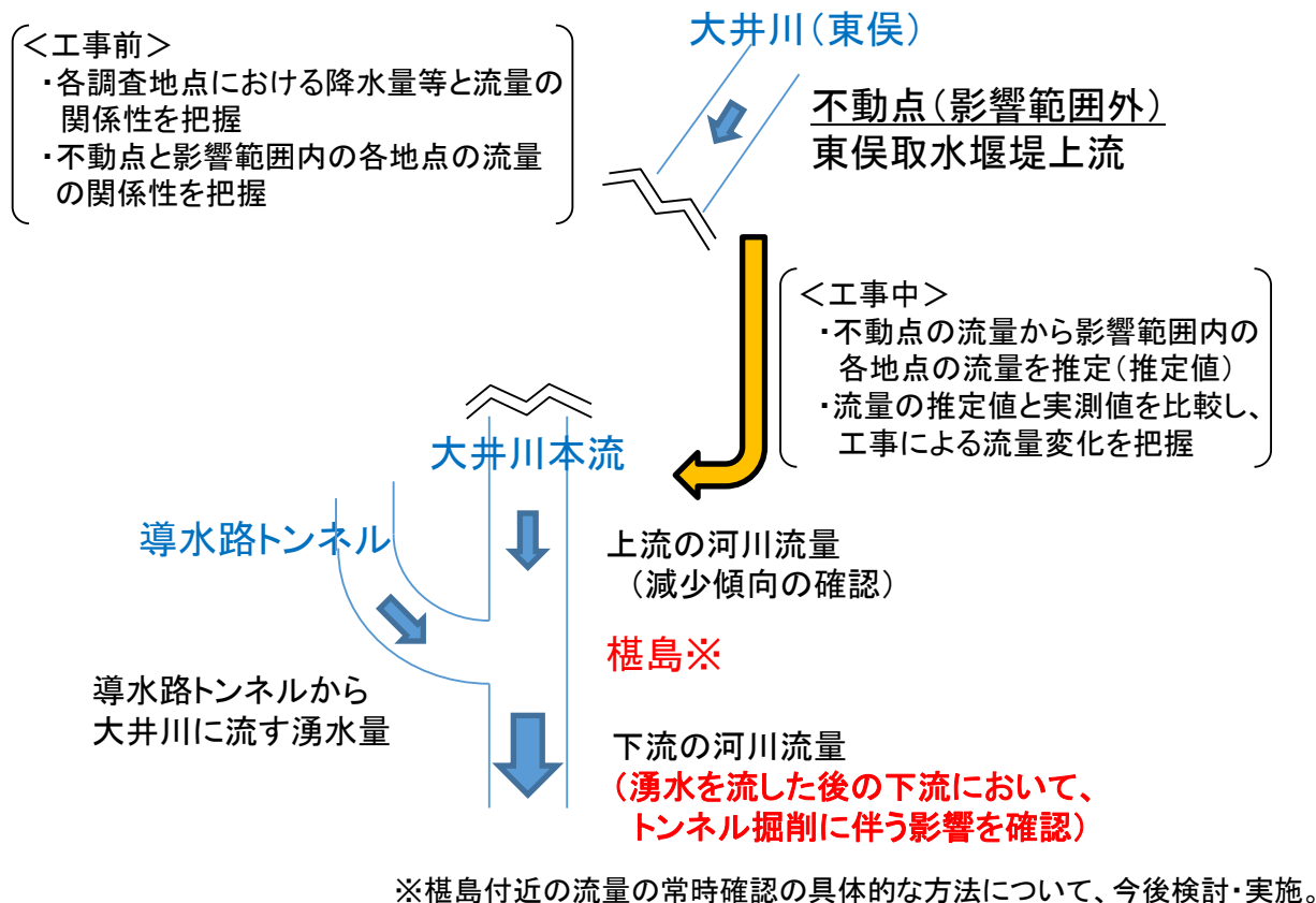
図 8.2 さわらじま 樫島下流における流量変化の把握イメージ
