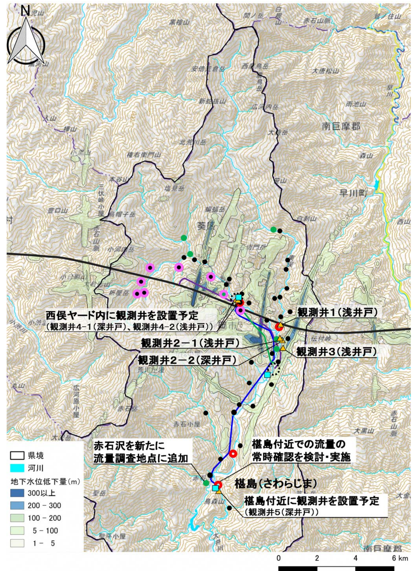
図 8.3 (1) 地下水位、河川等の流量 調査地点 (上流域)
