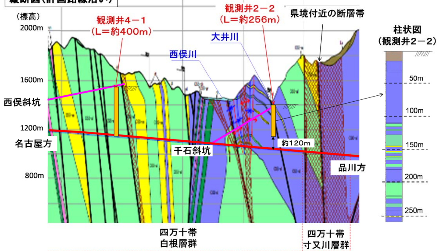
図 8.4 深井戸と本坑との位置関係
