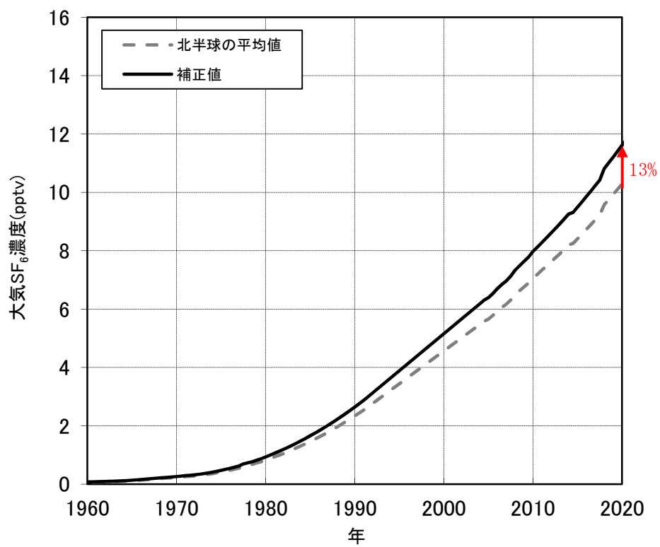
図 3-20 大気中の \text{SF}_6 濃度の経年変化曲線 (北半球平均値) の補正結果 : 渇水期調査
