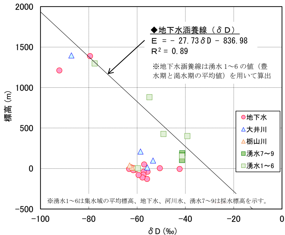
図 3-17 (1) 地下水涵養線 (δD) の算出結果：渇水期調査
