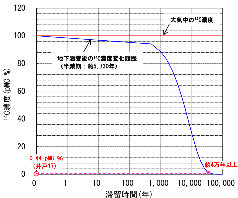
図 3-22 ^{14}\text{C} 濃度の経年変化曲線及び滞留時間の推定結果：渇水期調査
