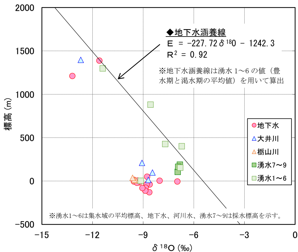
図 3-17 (2) 地下水涵養線 (δ¹⁸O) の算出結果：渇水期調査
