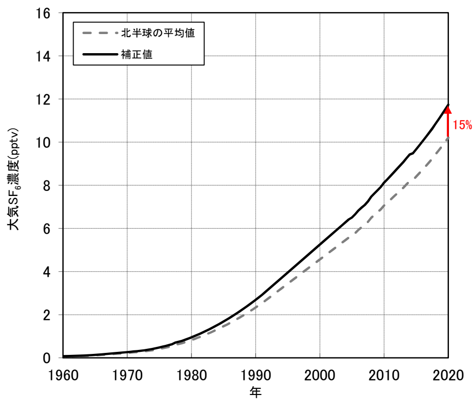
図 3-1 2 大気中の \text{SF}_6 濃度の経年変化曲線 (北半球平均値) の補正結果 : 豊水期調査
