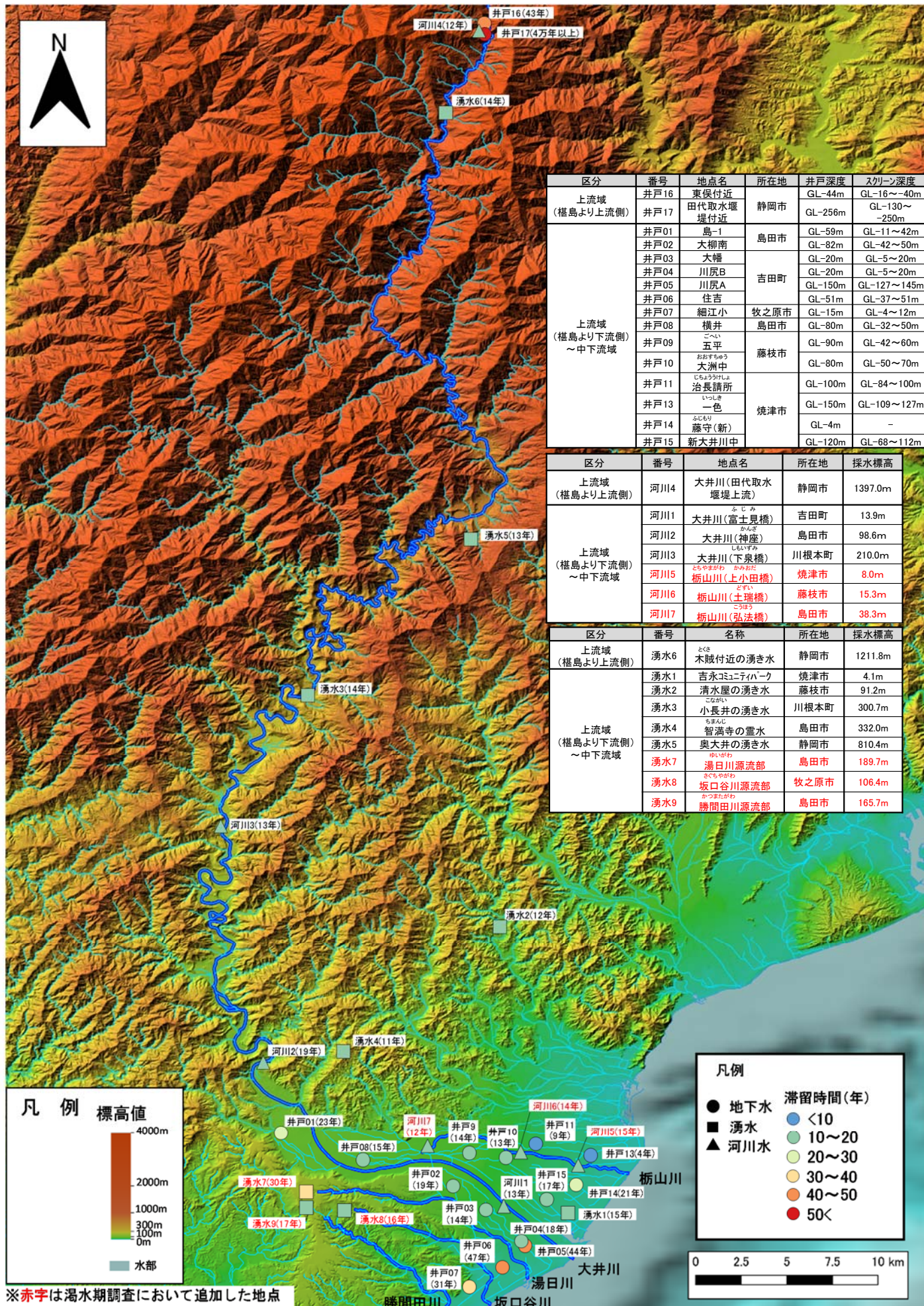
図 3-23 滞留時間推定結果の平面分布：湧水期調査
