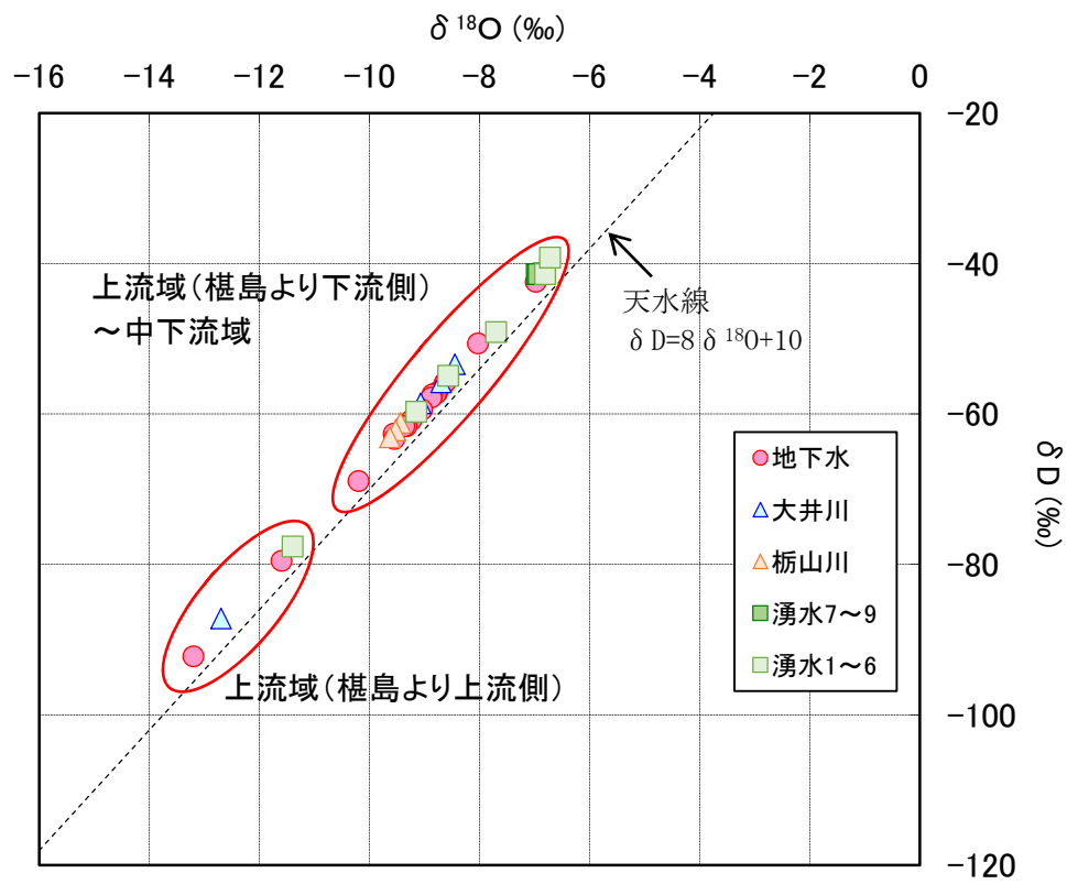
図 3-19 δダイヤグラムと天水線：渇水期調査
