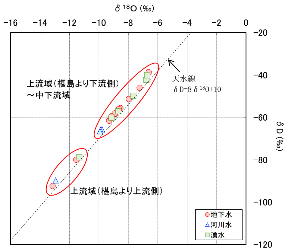
図 3-1 1 \delta ダイアグラムと天水線：豊水期調査
