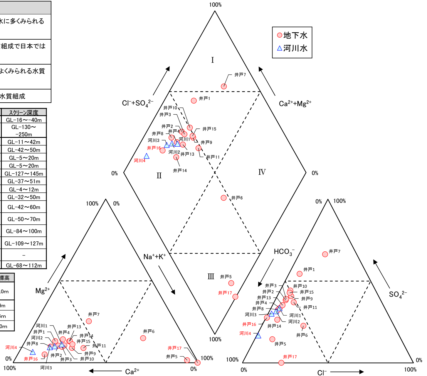
図 3-8 トリリニアダイアグラム：豊水期調査
