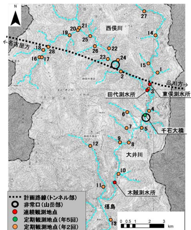
図 5-2 1 モデル検証で用いた観測地点
