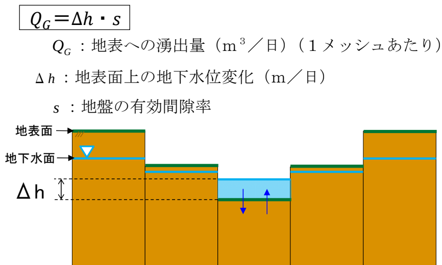
図 5-6 地表への湧出量の算出方法
