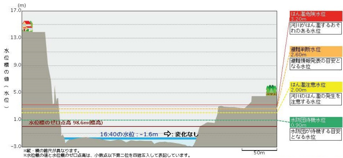
図 2.7 大井川（神座地点）の断面図
