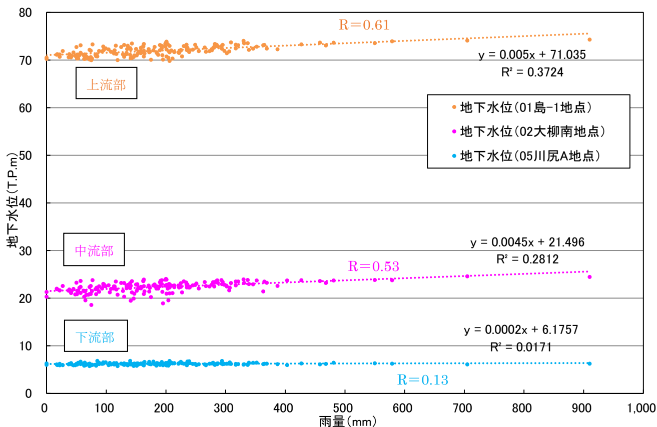
図 2.19 (1) 地下水位と島田観測所雨量の相関関係
