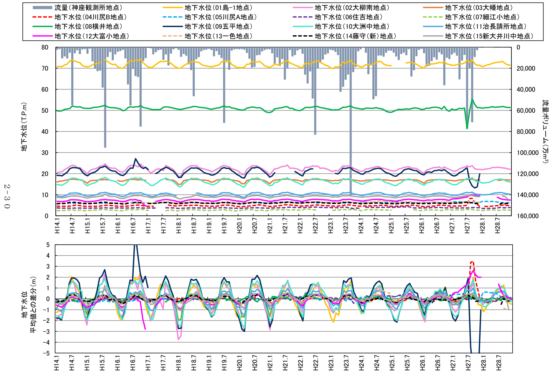
図 2.20 地下水位と神座地点流量の経年変化 (H14~H28)
