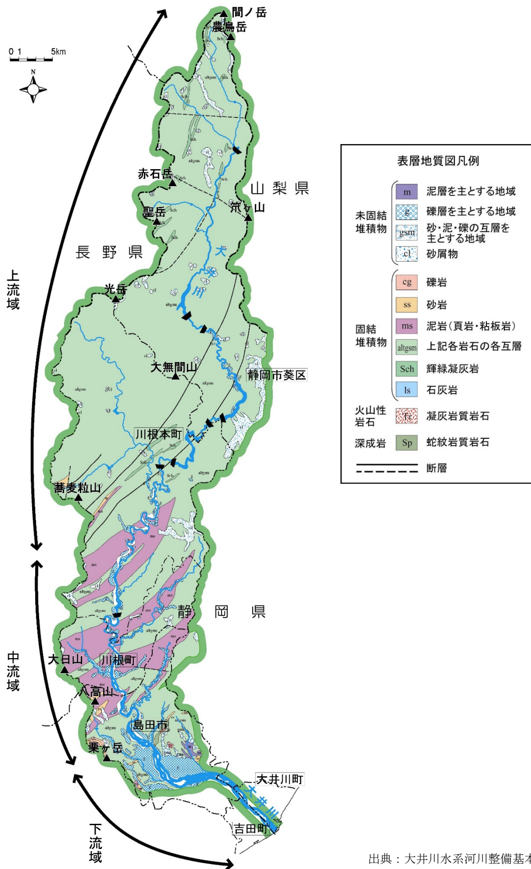
図 2.4 大井川流域の地質図
