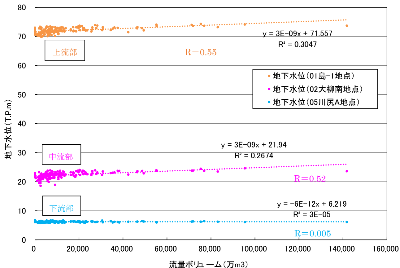
図 2.21 (1) 地下水位と神座地点流量の相関関係
