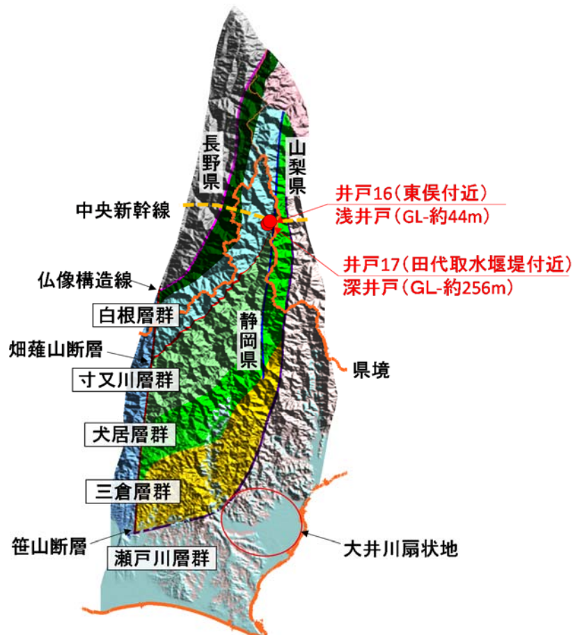
図 2.24 大井川流域の地層分布と上流域（榎島以北）の観測井の位置図
