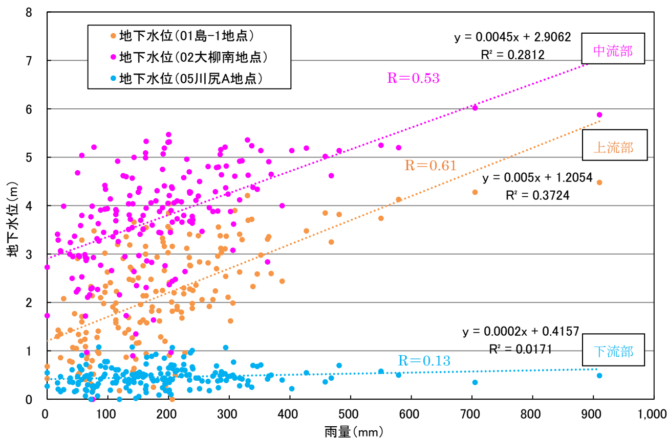
図 2.19 (2) 地下水位と島田観測所雨量の相関関係 (拡大図)
