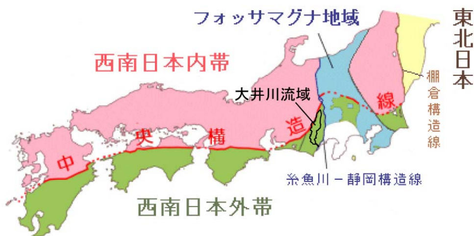
図 2.3 中央構造線と糸魚川－静岡構造線の位置
