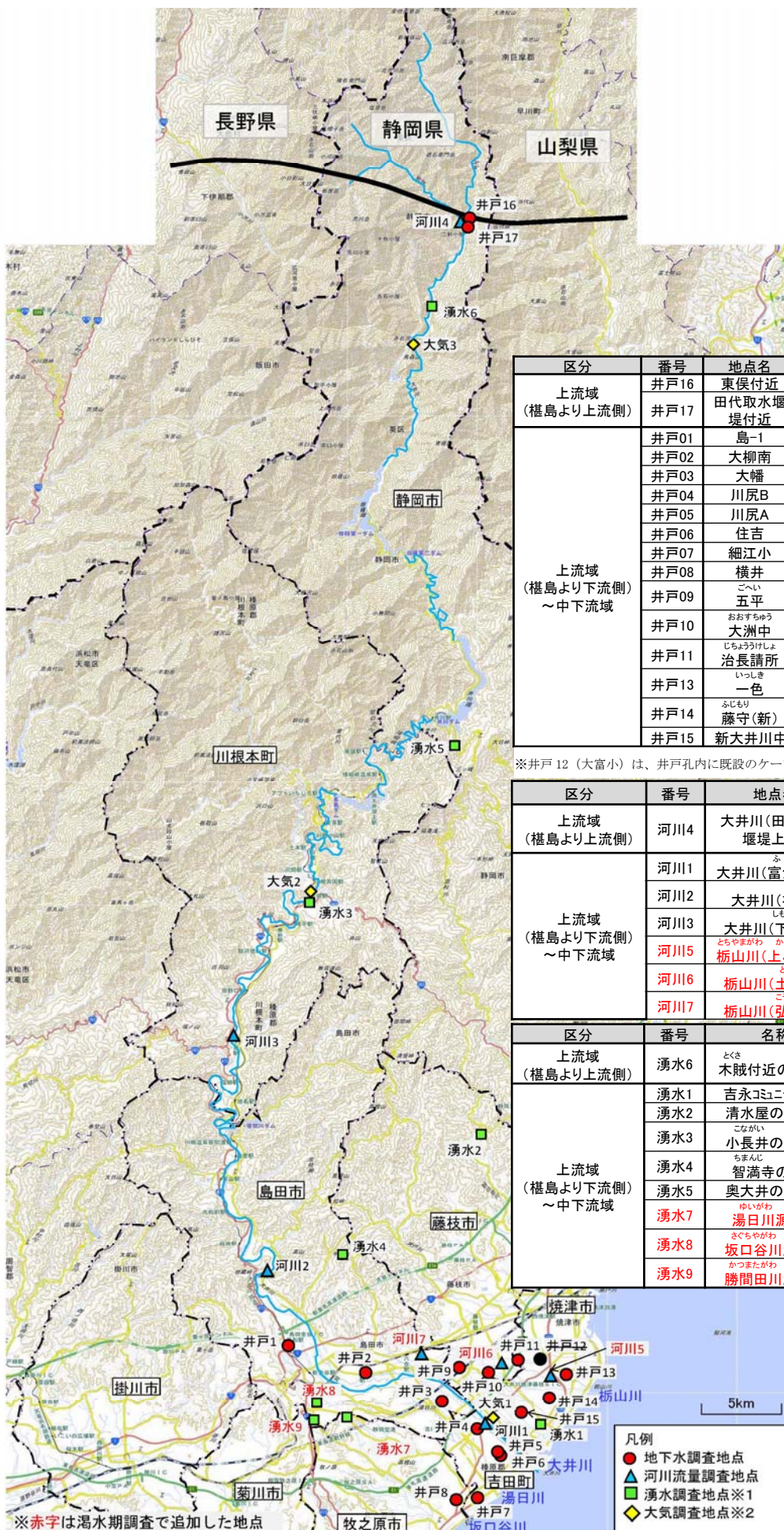
図 2.27 (1) 成分分析の計測地点(湧水期調査)
