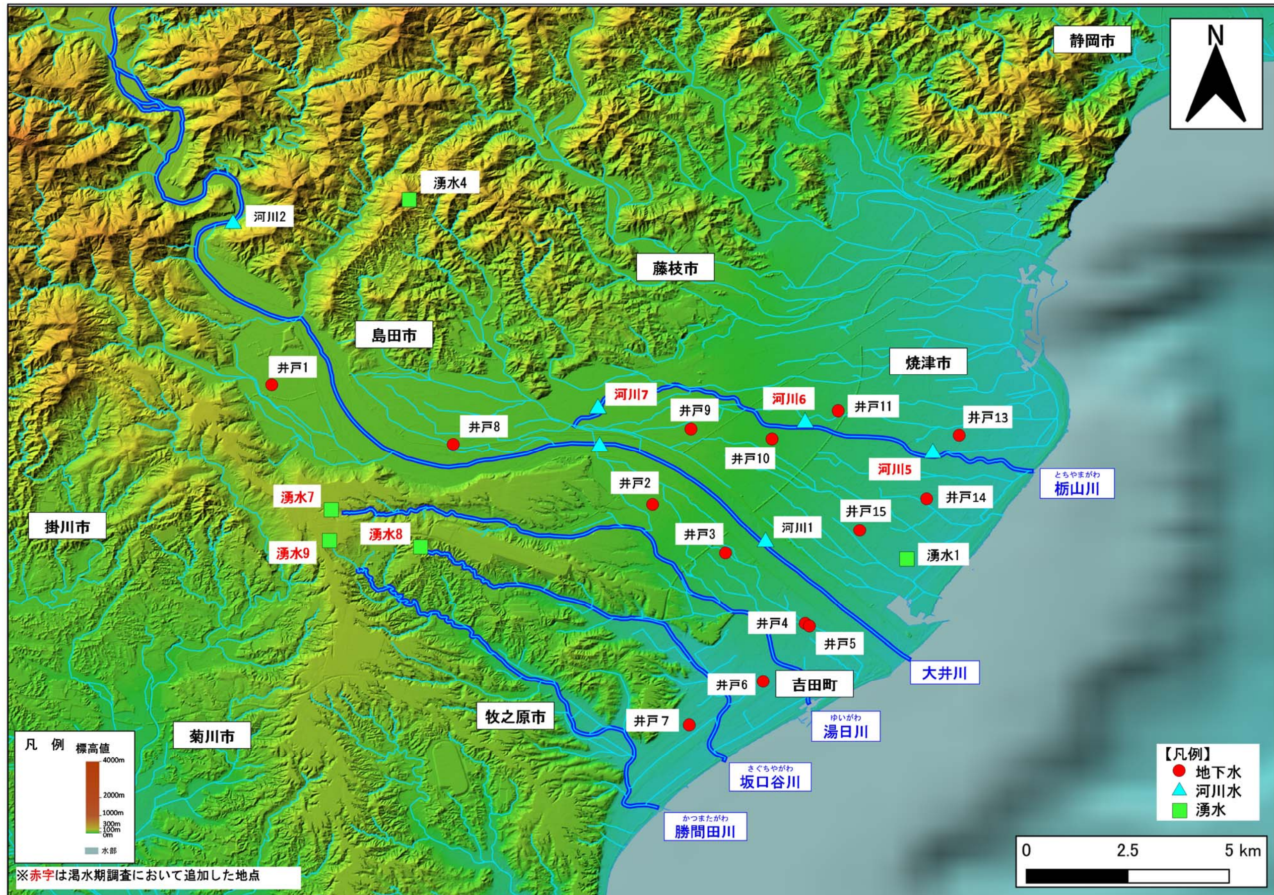
図 2.27 (2) 成分分析の計測地点（渇水期調査）：下流域拡大図
