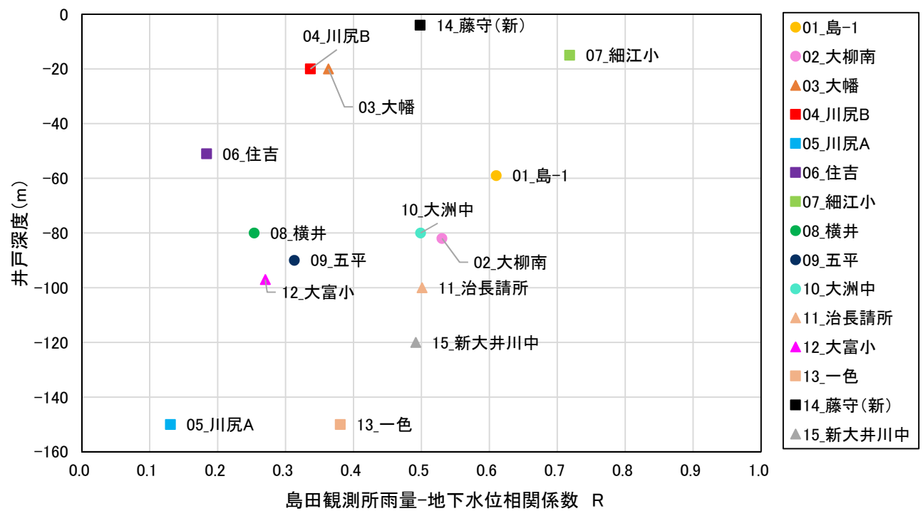
図 2.22 井戸深度と地下水位・島田観測所雨量の相関関係
