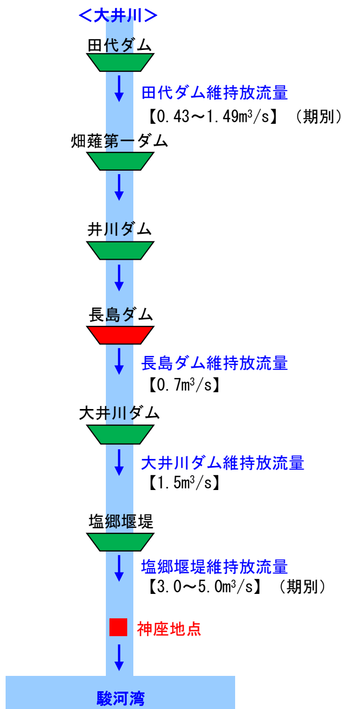
図 2.8 維持放流量模式図
