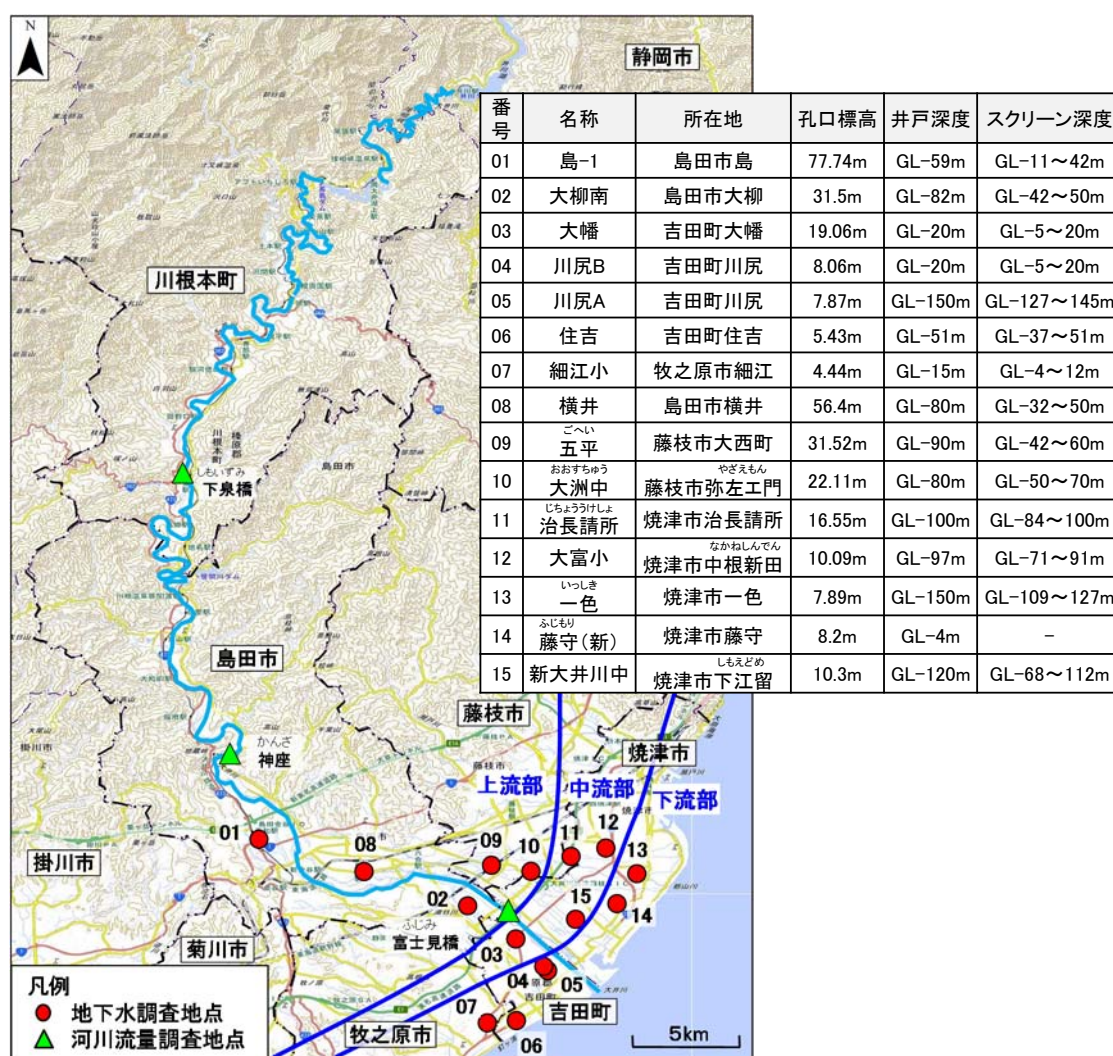
図 2.14 地下水の水位 調査地点図（大井川下流域）
