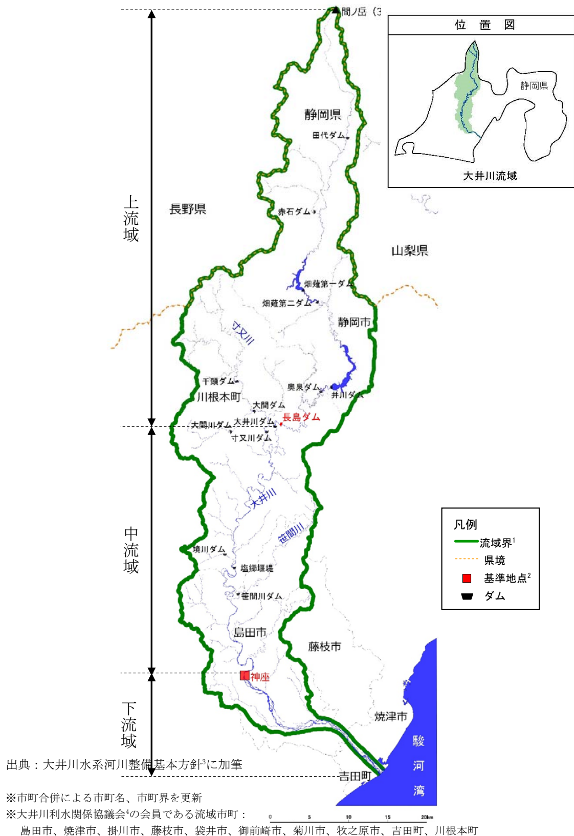
図 2.1 大井川流域図
