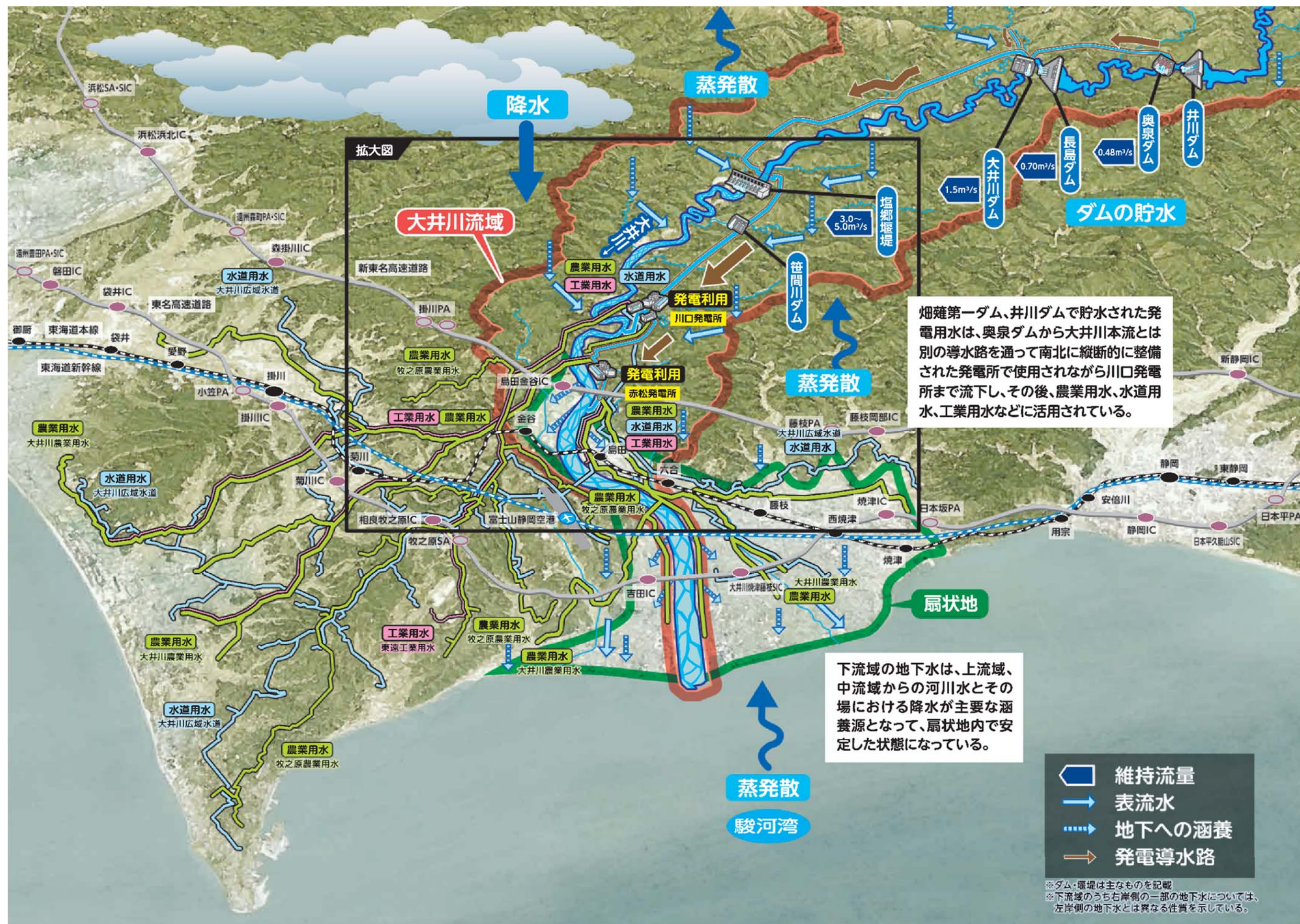
図 2.30 大井川流域の水循環の概要図 <鳥瞰図・井川ダム下流側>
