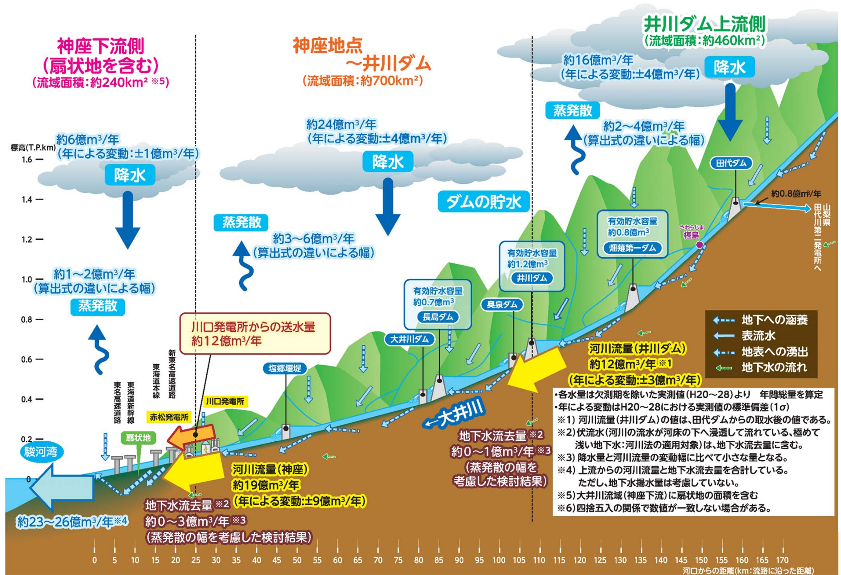
図 2.32 大井川流域の水循環の概要図 <現状の水循環量>
