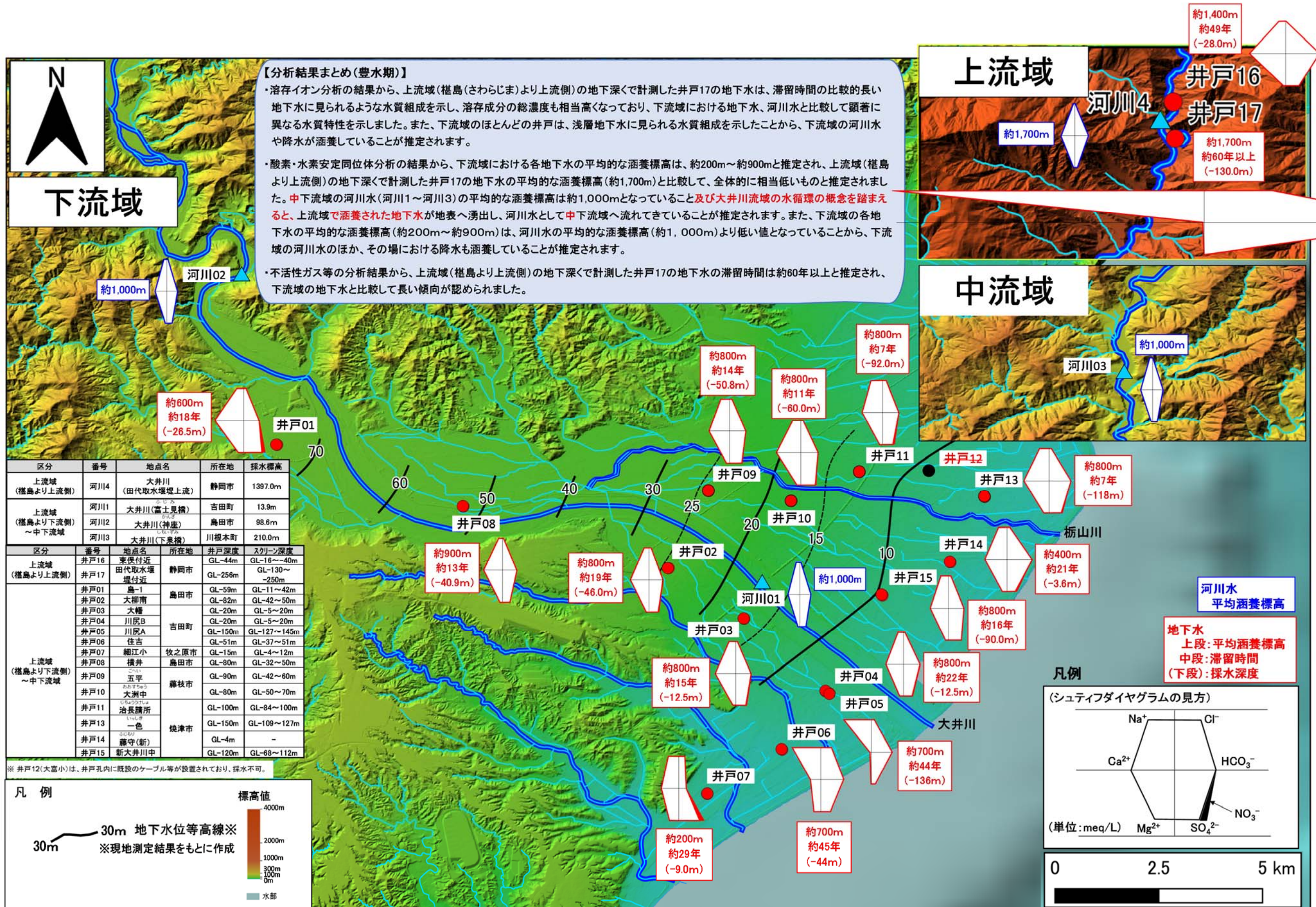
図 2.26 成分分析結果まとめ(豊水期調査)
