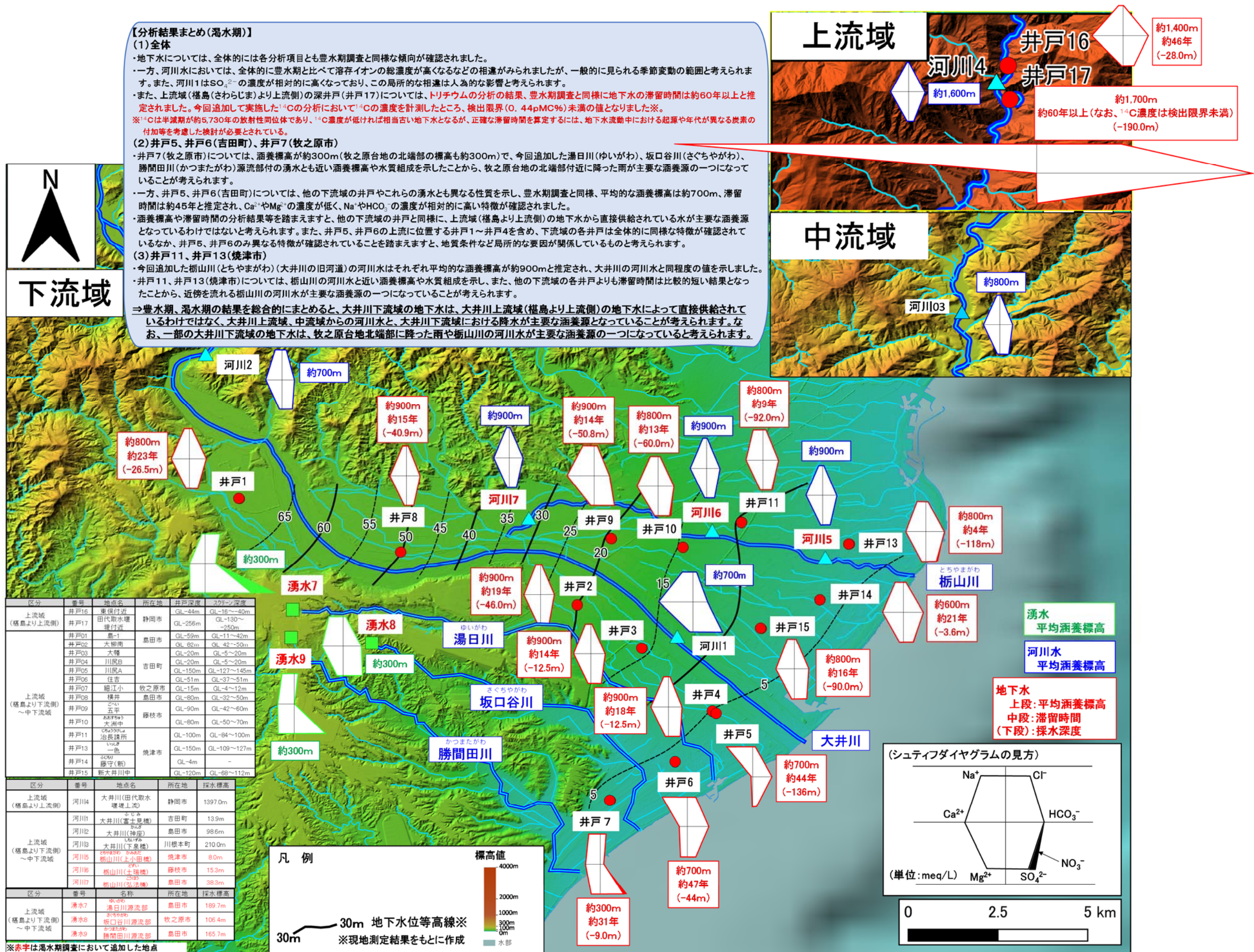
図 2.28 成分分析結果まとめ(渇水期調査)
