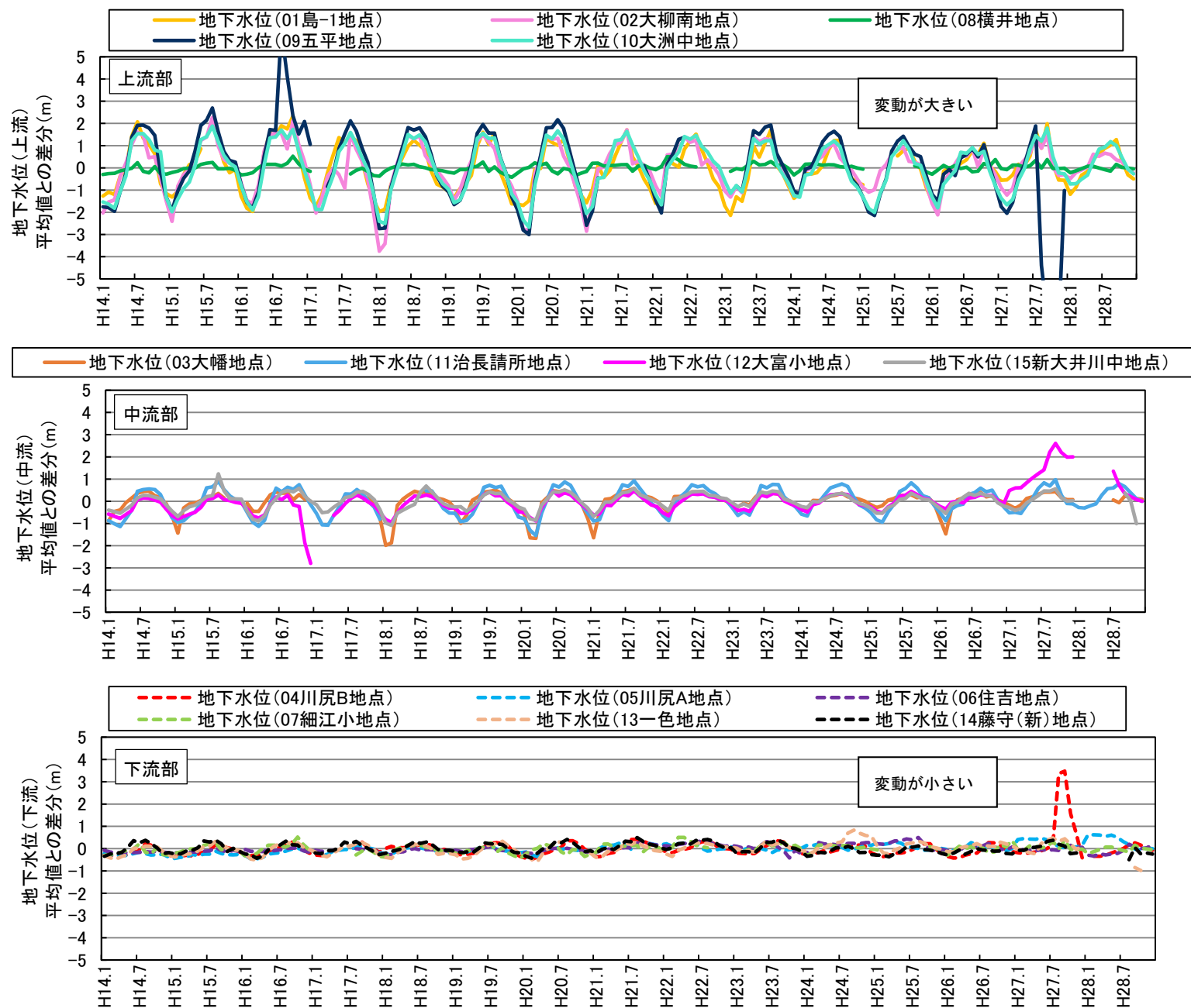
図 2.18 地下水位の平均値との差分 (H14～H28)
