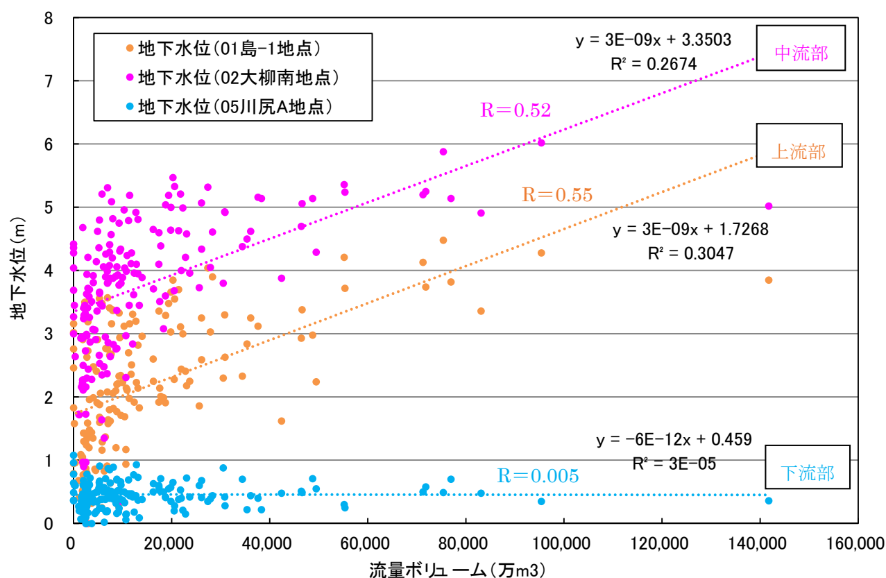
図 2.21 (1) 地下水位と神座地点流量の相関関係
