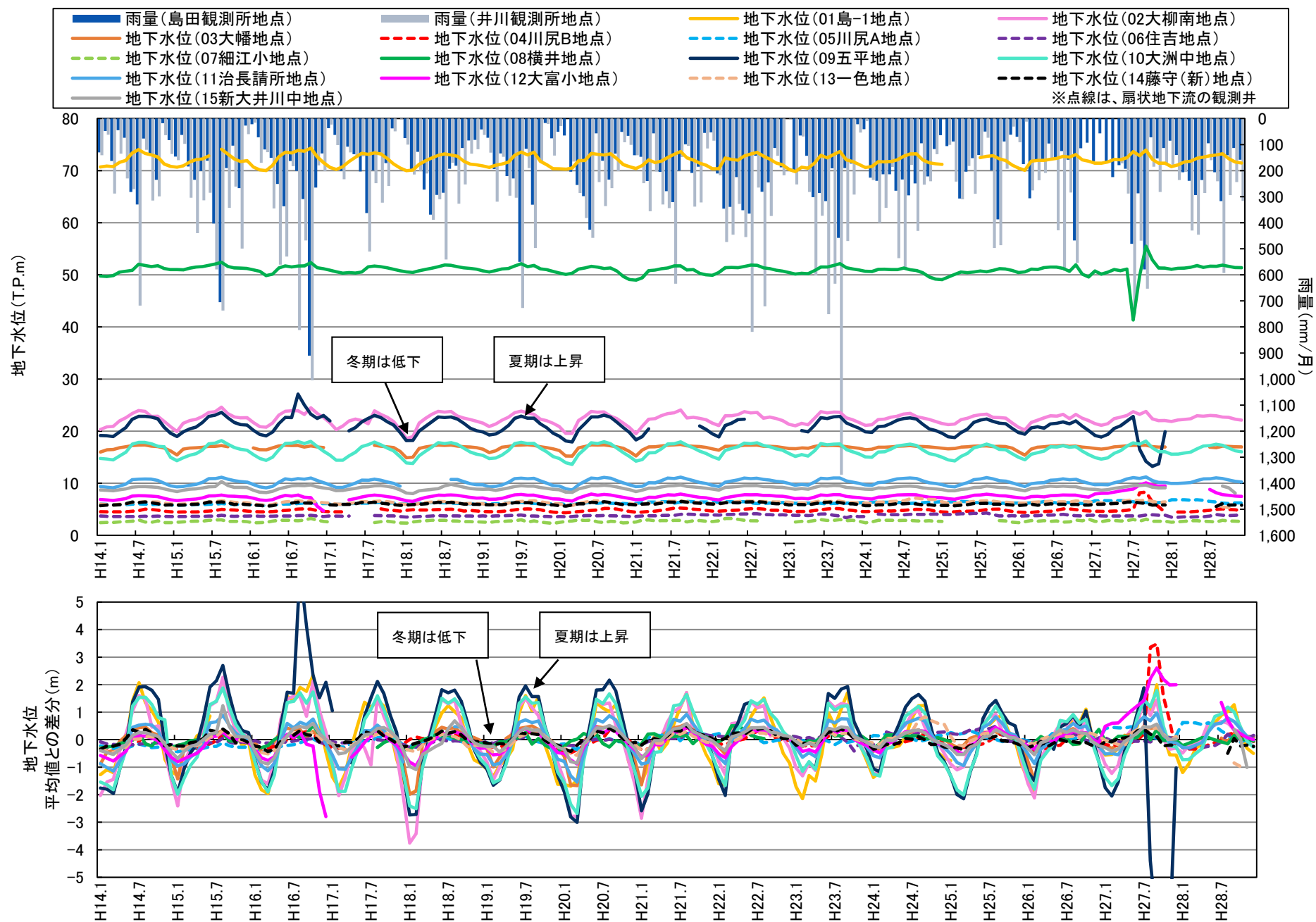
図 2.17 地下水位と降水量の経年変化 (H14～H28)
