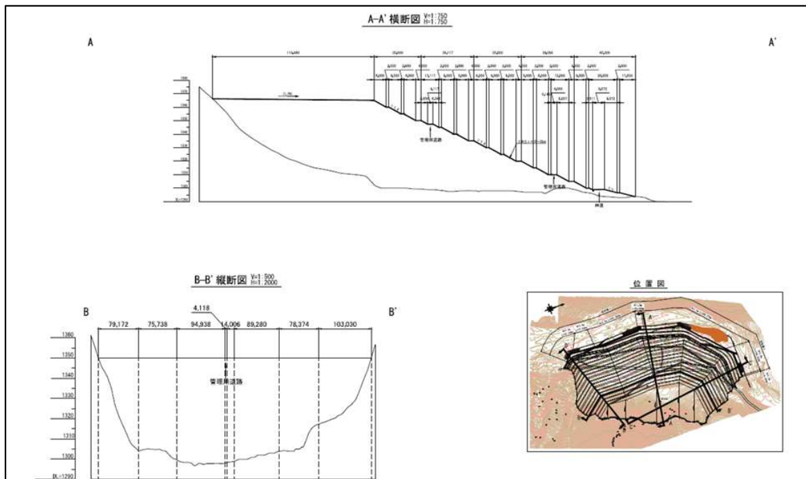
図5 ツバク口発生土置き場 縦横断面図
