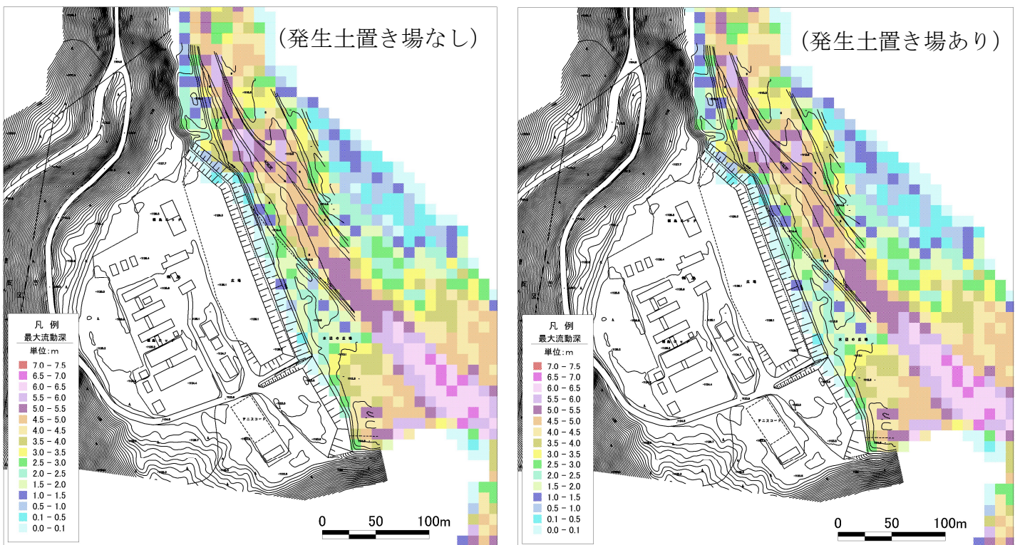
図18 河道閉塞決壊時の榎島ロッヂ付近での最大水深予測結果
