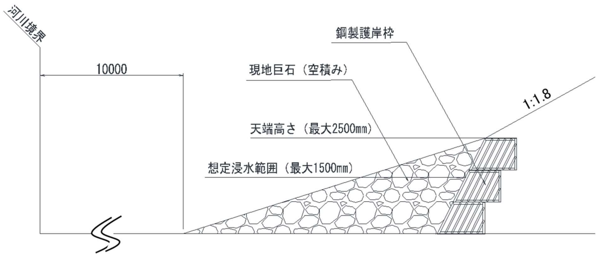
図6 盛土のり尻詳細図
