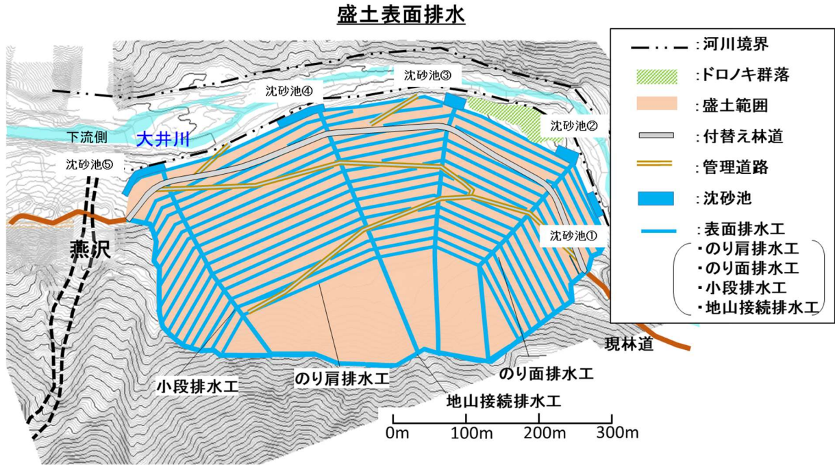
図4 ツバク口発生土置き場 計画平面図
