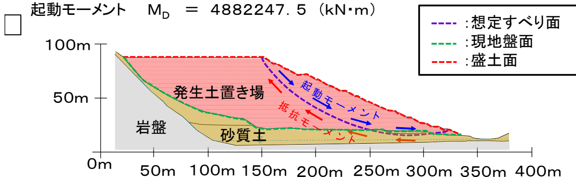
図7 盛土円弧すべり安定検討（ツバクロ発生土置き場）
