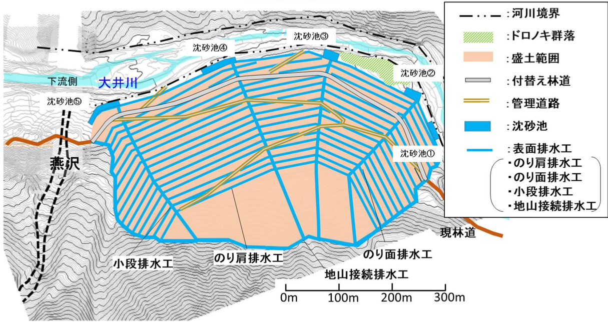
図9 盛土排水計画平面図
