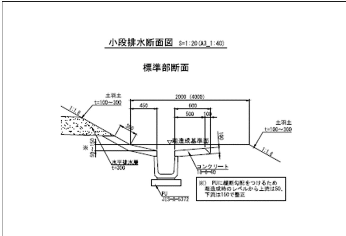
図10 小段排水工詳細図
