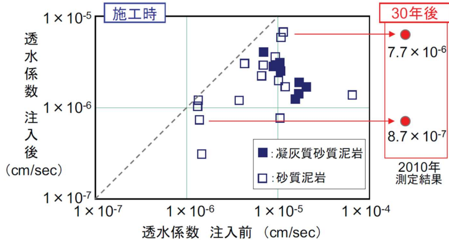
図 3-19 透水係数分布図 (施工前と施工後の比較) 7
