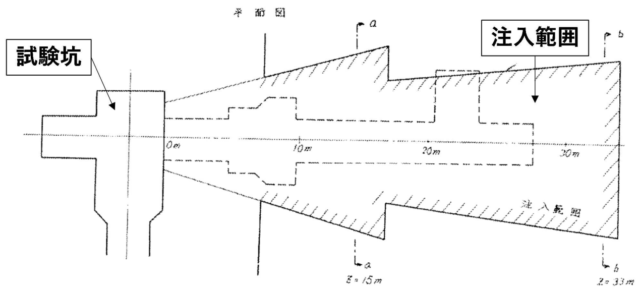
図 3-3 止水注入（薬液注入）の平面図（JR東海一部追記） 1
