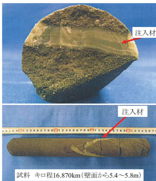
図 3-15 施工 30 年後に採取した直後の試料の状況 7
