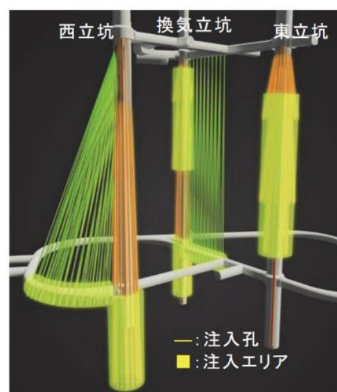
図 3-13 グラウト改良範囲(立坑) 6
