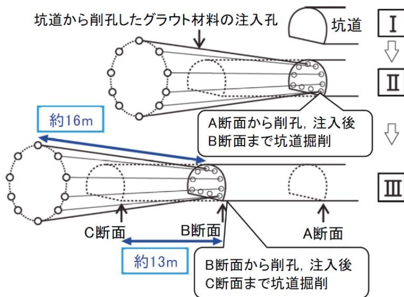
図 3-11 プレグラウティングと坑道掘削の標準的な施工パターン 5
