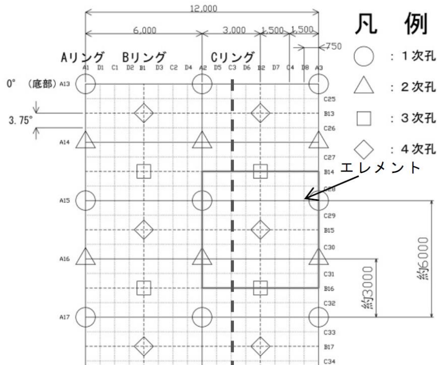
図 3-8 孔配置 (平面展開図) 2
