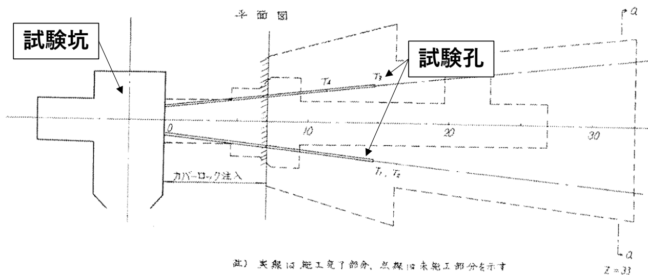
図 3-2 薬液注入前の自然地山の透水性を調査した際の試験孔 (平面図) (J R 東海一部追記) 1
