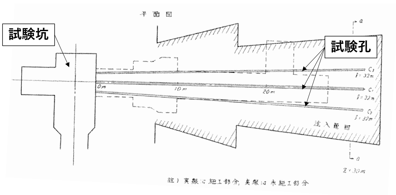
図 3-4 薬液注入後の透水性を調査した際の試験孔（平面図） （JR東海一部追記） 1
