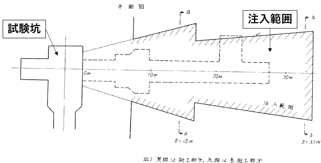
図 3-3 止水注入 (薬液注入) の平面図 (J R 東海一部追記) 1
