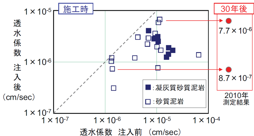
図 3-19 透水係数分布図（施工前と施工後の比較） 7
