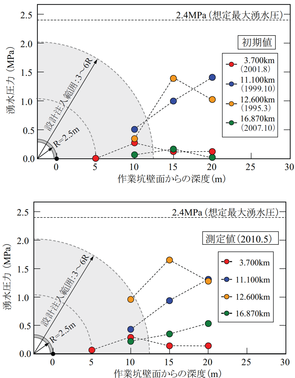
図 3-17 注入域における湧水圧の分布 (2010.5 時点) 7
