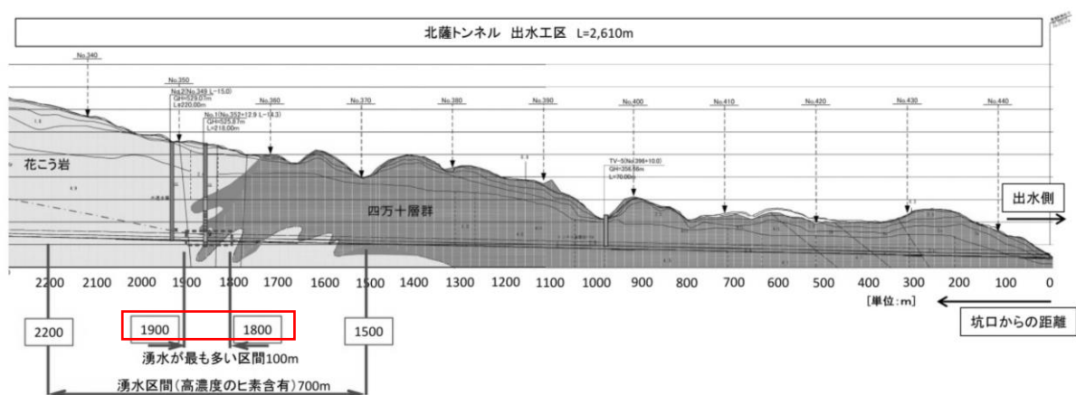
図 3-5 北薩トンネルの地質縦断図（JR 東海一部加筆） 2
