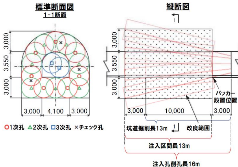
図 3-10 プレグラウティング孔の標準的な配置（単位：mm） 5
