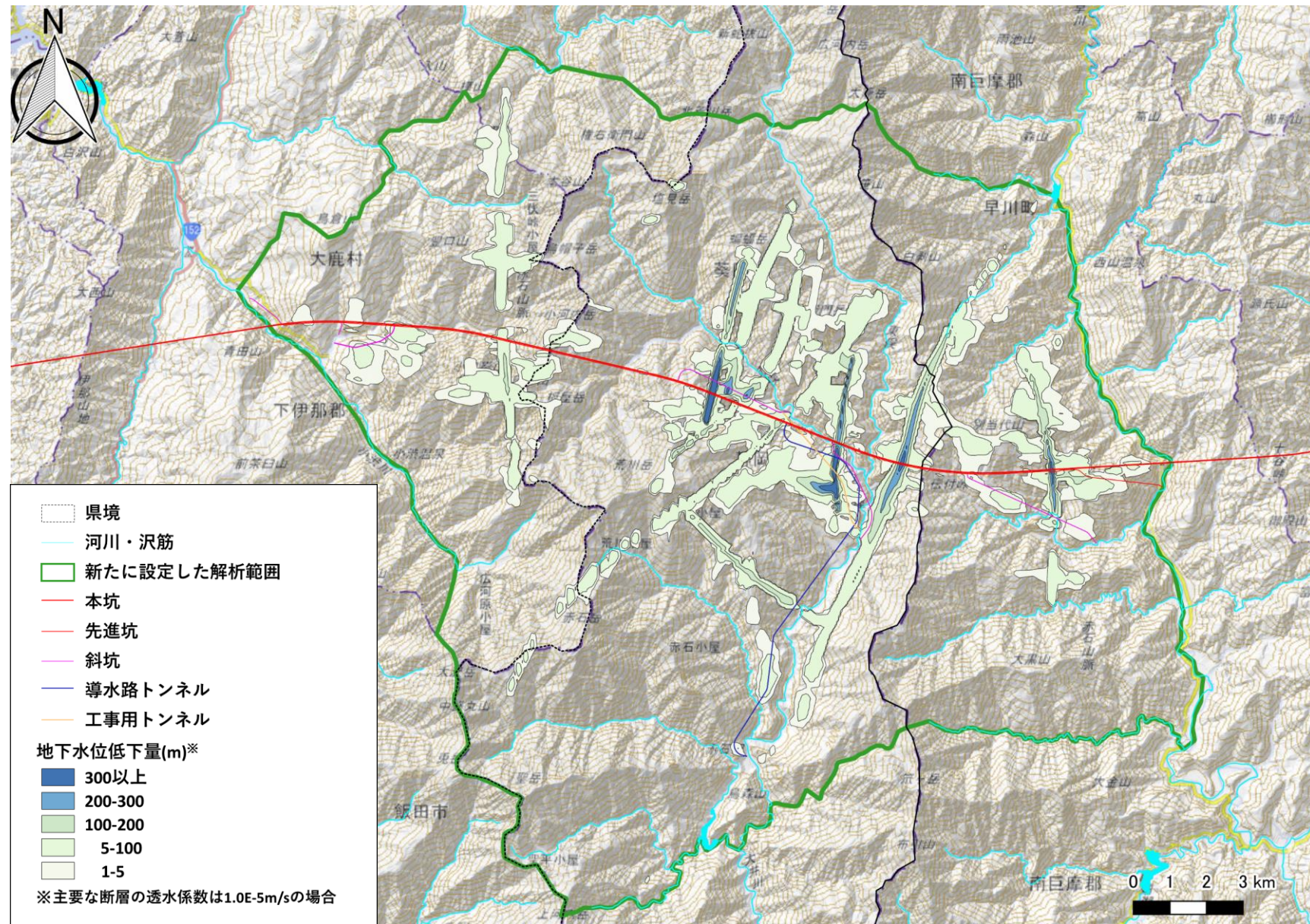
図 3.20 新たに設定した解析範囲と現状の静岡市モデル (断層部の透水係数 1.0E-5 (m/s))での地下水位低下量図
