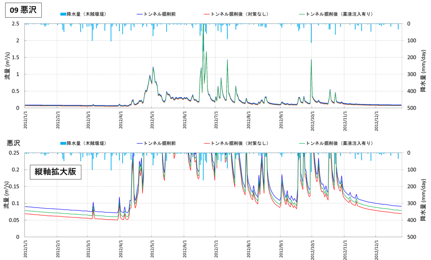
図 3.41 悪沢の流量変化 (非定常解析)
