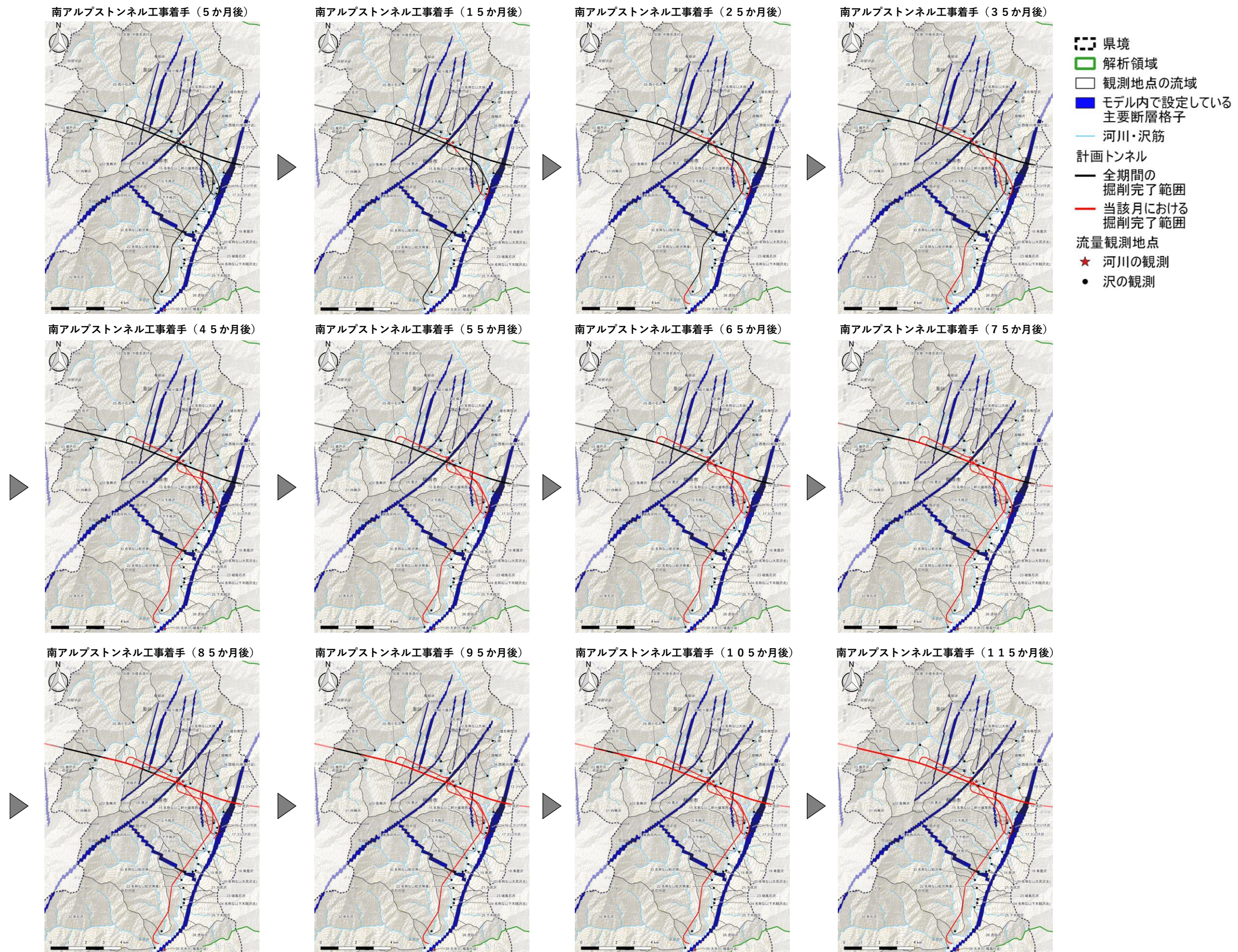
図 3.50 解析上想定した南アルプストンネル工事着手後のトンネル掘削の進行状況
