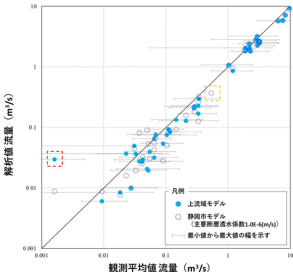
図 3.25 上流域モデルの解析値と観測平均値の流量の比較 (静岡市モデル (主要断層透水係数 1.0\text{E-}6(\text{m/s}) ) の結果を併記)
