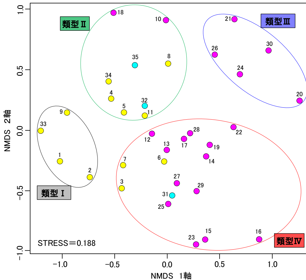
図 3.82 PCA と NMDS による分析結果まとめ
