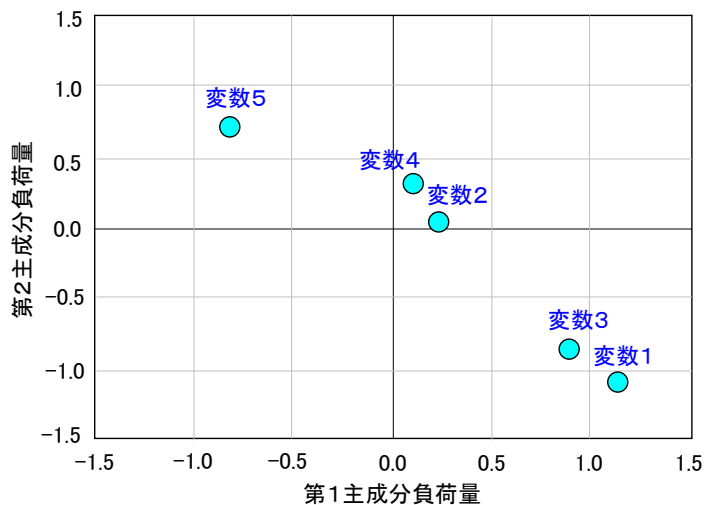
図 3.7 2 主成分分析結果の整理イメージ
