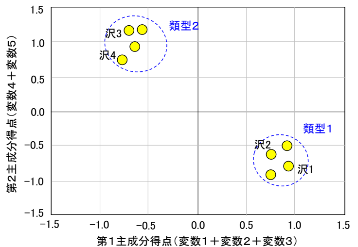
図 3.7 2 主成分分析結果の整理イメージ
