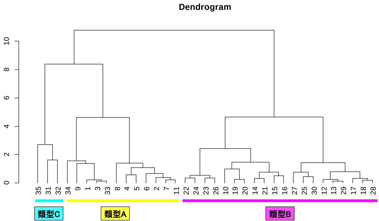
図 3.78 デンドログラム (PCA)
