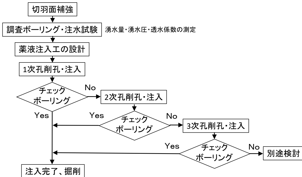
図 3.87 薬液注入工の一般的な施工フロー
