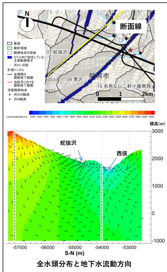
トンネル掘削前
