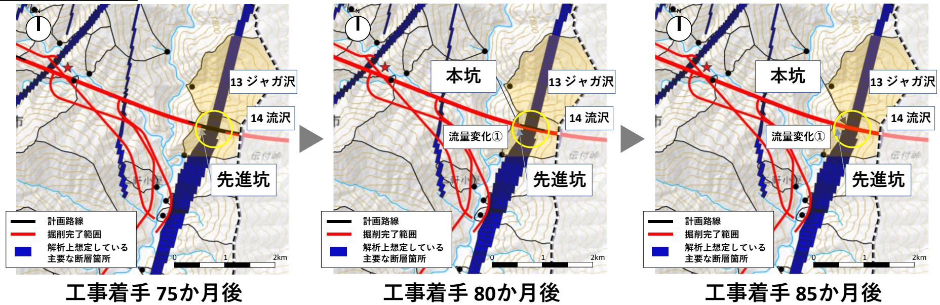
図 3.60 南アルプストンネル工事着手後のトンネル掘削の進行状況 (ジャガ沢、流沢周辺：流量変化①)
