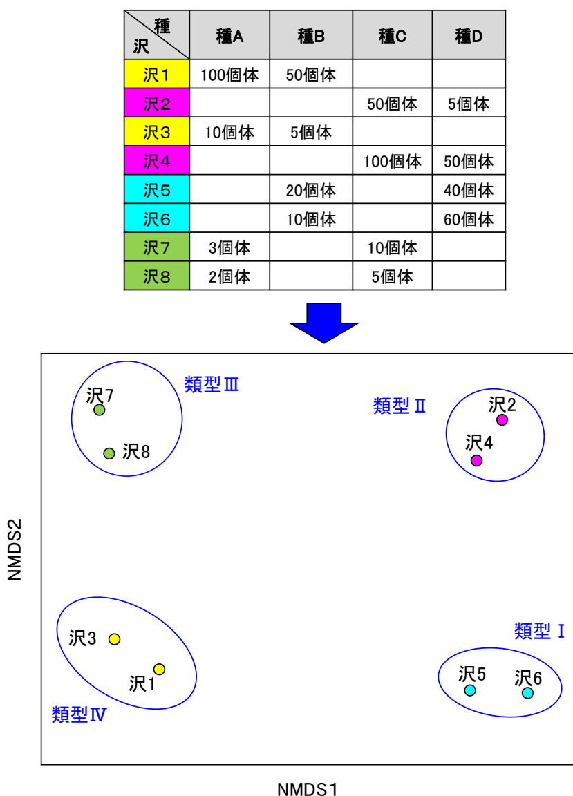
図 3.73 NMDS による分析のイメージ
