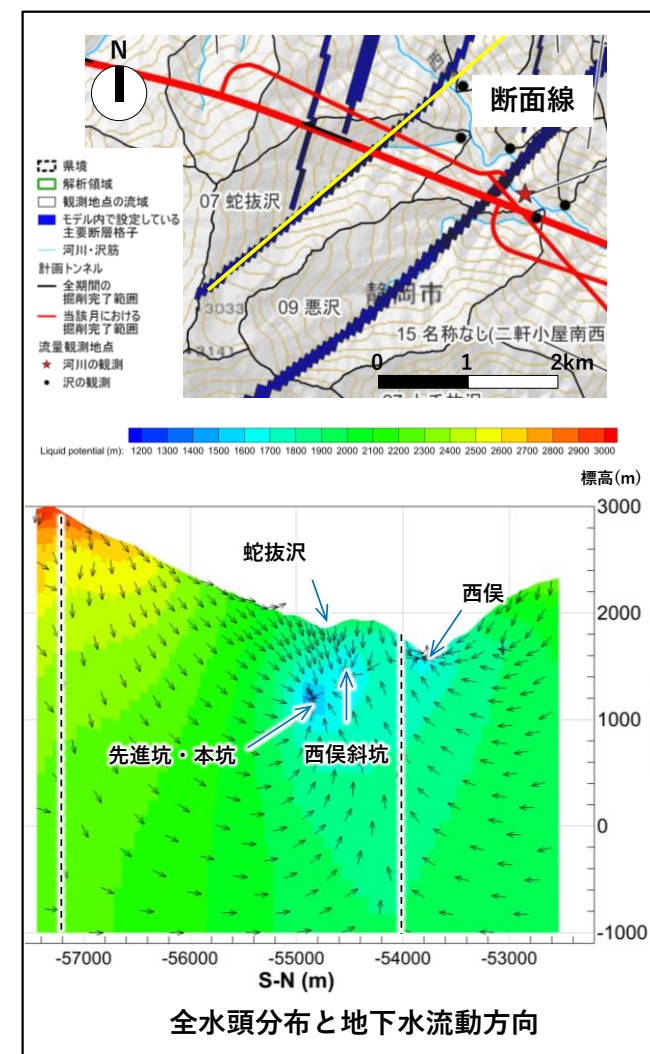
トンネル掘削90か月後
