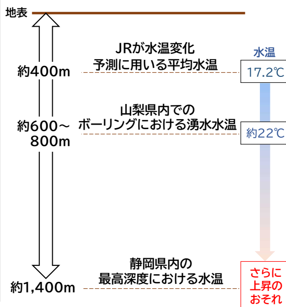
トンネル湧水の水温変化(想定イメージ図)
