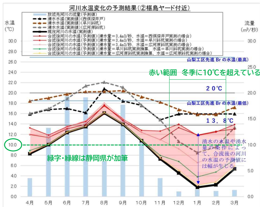
工事完了後の河川水温変化の予測結果
