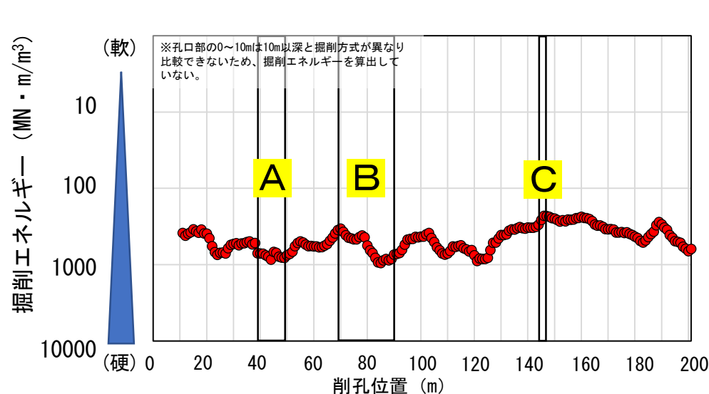
図-1 掘削エネルギーグラフ 削孔位置（0m～201m）（県境まで501m～300m）
