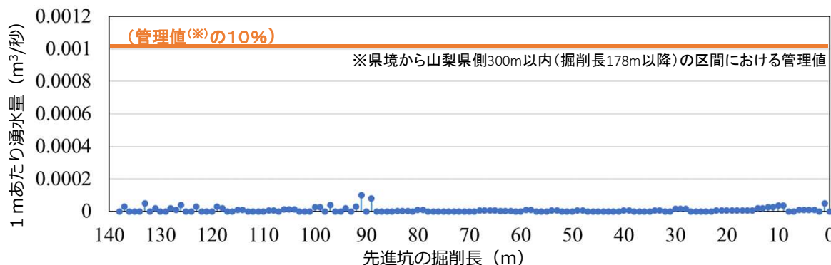
先進坑の進捗と1mあたり湧水量の推移
