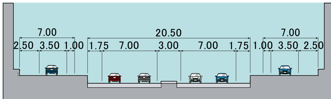
④堀割部
