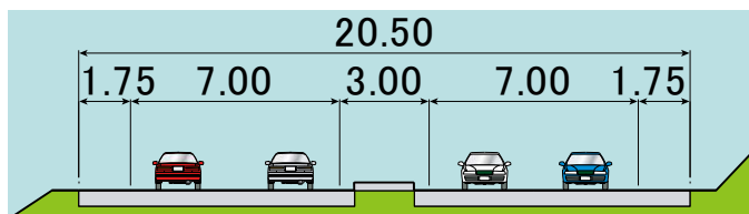
①土工部
