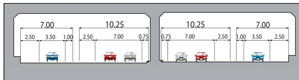
③トンネル部(ボックストンネル)
