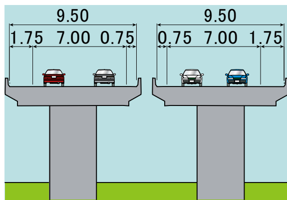
②橋梁部
