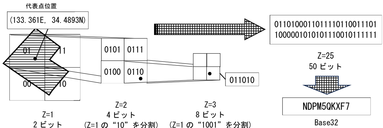
図 1 GeoHash 概要
