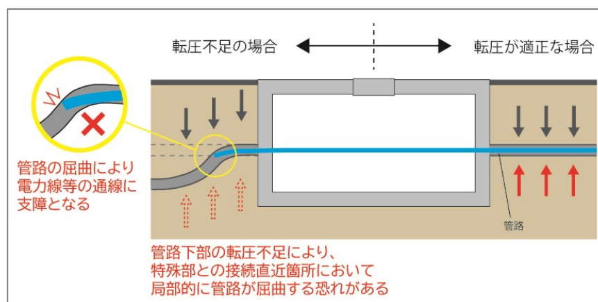
【図】 角型 FEP 管における屈曲の一例
