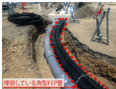
【写真】 多治見駅南地区の様子 (交通広場歩道部に曲げ半径約 5m で埋設)
