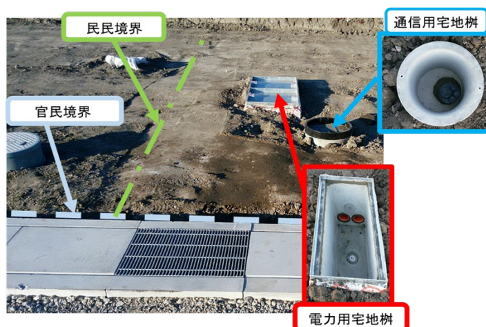
【写真】 各種宅地枿の施工の様子
