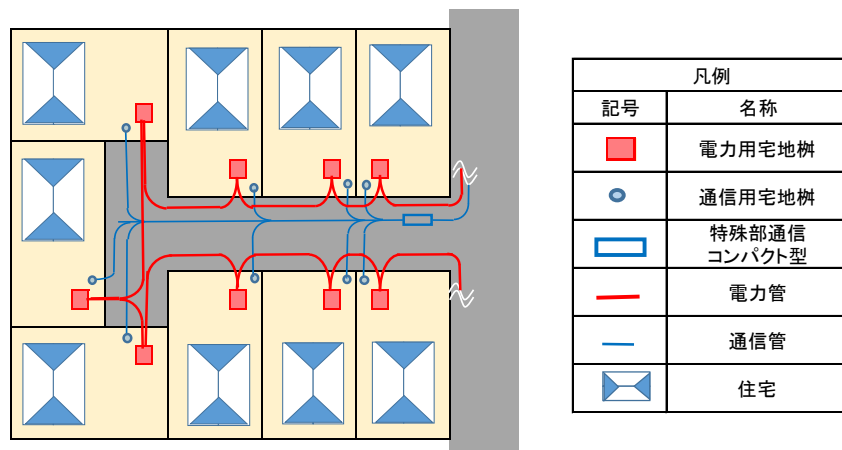
【図】 宅地枿等の配線イメージ
