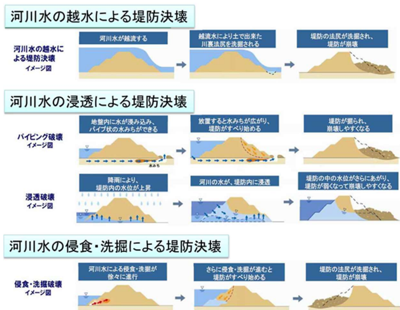
図 1-2 代表的な堤防決壊のメカニズム
