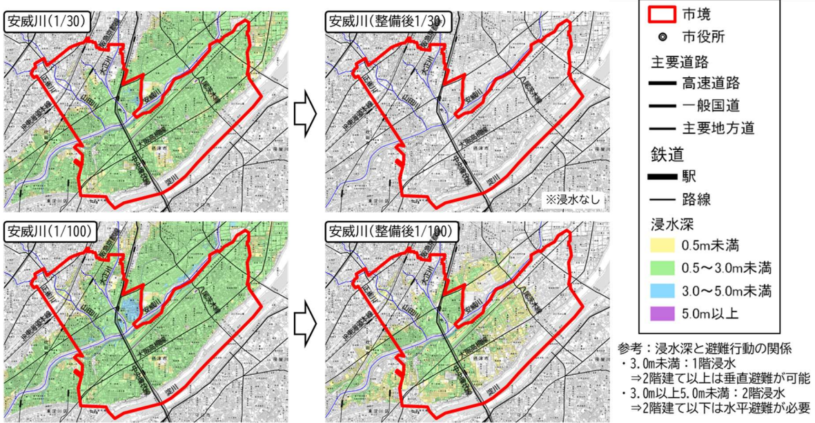
図 1-17 施設整備前後の浸水想定の例
