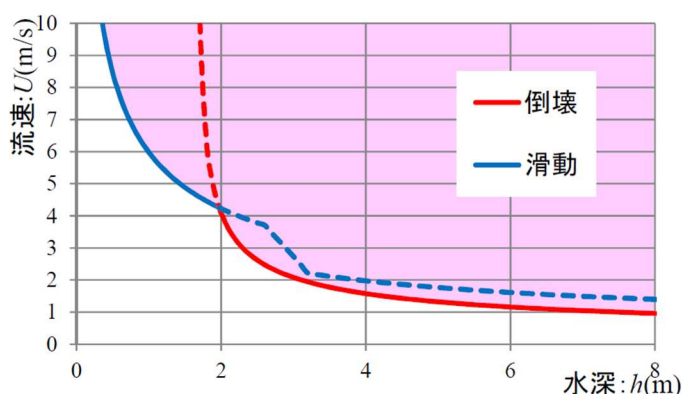
図 1-3 木造家屋の倒壊等に係る流速・水深の関係例 (モデル的な家屋、荷重条件等を想定しての試算の一例)
