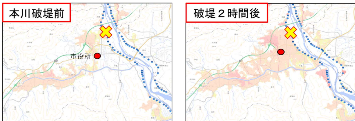
図 1-19 内外水統合型浸水解析の活用例
