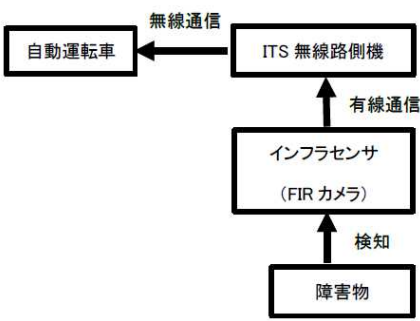
図 4: 地上側インフラセンサのシステム構成および設置の様子
