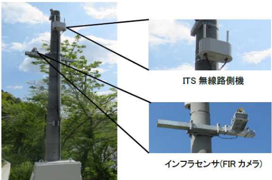
図 4: 地上側インフラセンサのシステム構成および設置の様子
