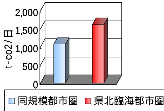
図 1-29 CO 2 排出量
