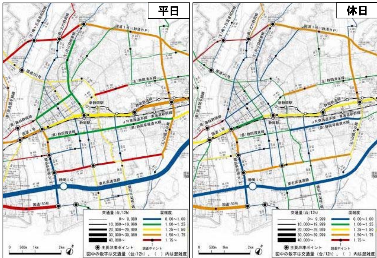
図4-21 静岡都心地区の交通量および混雑度
