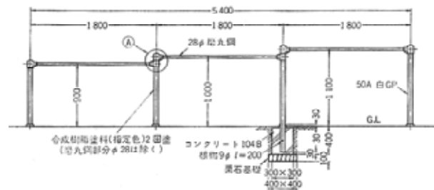
鉄棒の例【出典：造園ハンドブック】
