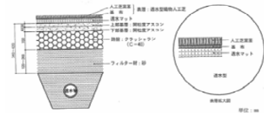
図面-41 透水性人工芝舗装断面図
