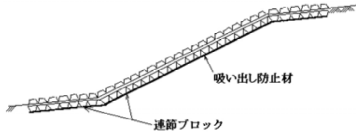
連節ブロック張の例【出典：改訂3版土木施工の実際と解説】
