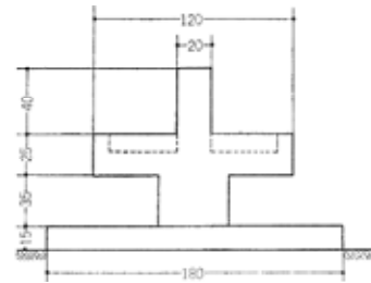
手洗い場の例【出典：造園ハンドブック】
