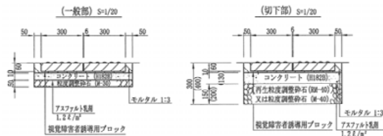
視覚障害者誘導用ブロックの例【出典：東京都建設局標準構造図集】
