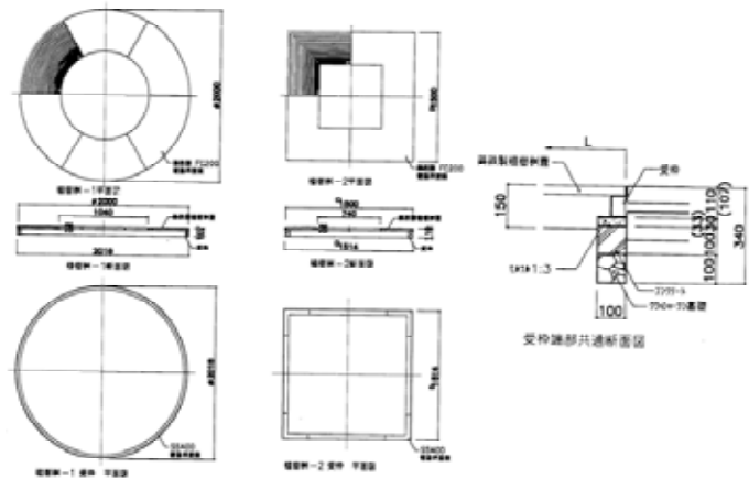
根囲い保護の例【出典：都市公園技術標準解説書平成22年度版】
