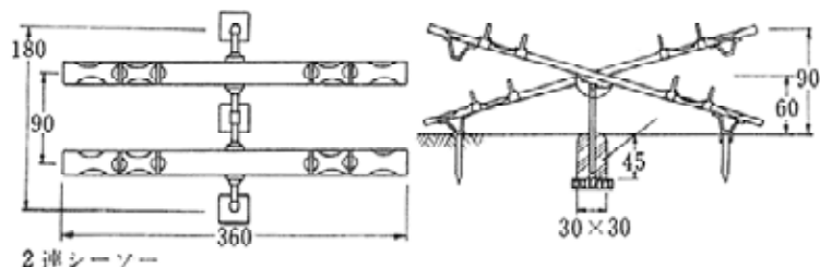
シーソーの例【出典：造園ハンドブック】
