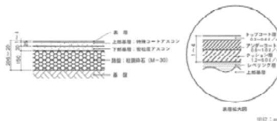
図面-29 アクリル樹脂系舗装断面図
