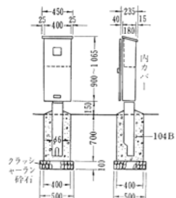
分電盤の例【出典：造園ハンドブック】
