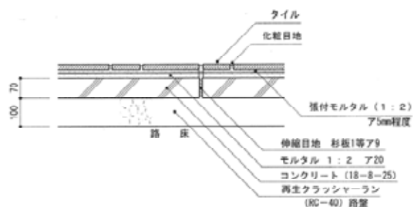
タイル舗装の例【出典：造園施設標準設計図集 平成19年】
