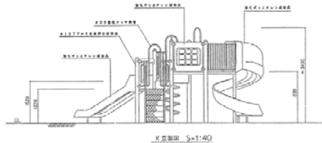
複合遊具の例
