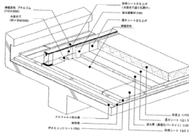
人工地盤排水層の例【出典：都市公園技術標準解説書（平成22年度版）】
