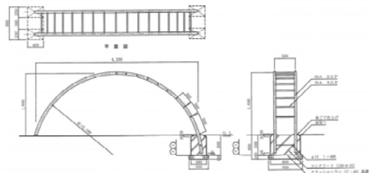
ラダーの例【出典：造園施設設計資料集】
