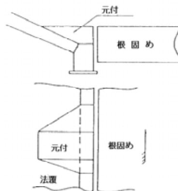
元付の例【出典：北陸地方整備局設計要領 河川編】
