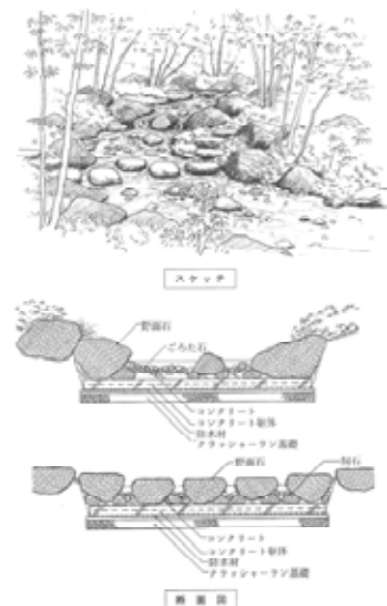
石組の例【出典：ランドスケープの修景石工事マニュアル】
