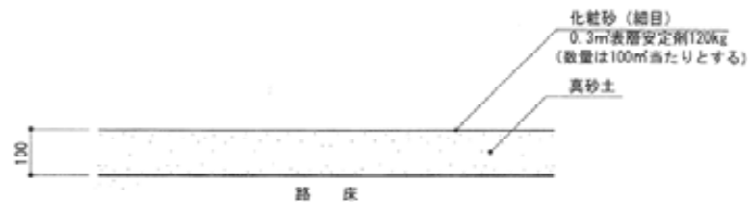
土舗装の例【出典：造園施設標準設計図集 平成19年】
