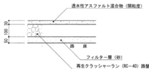
透水性アスファルト舗装の例【出典：造園施設標準設計図集 平成19年】
