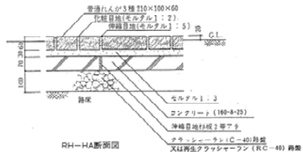
レンガ舗装の例【出典：造園施設標準設計図集 平成6年】
