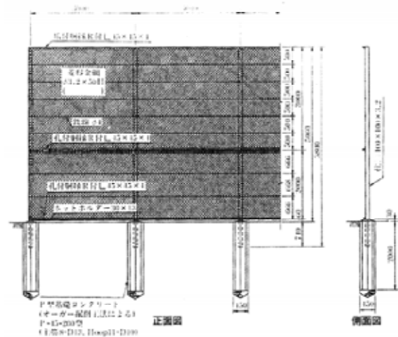
高尺ネットフェンスの例
