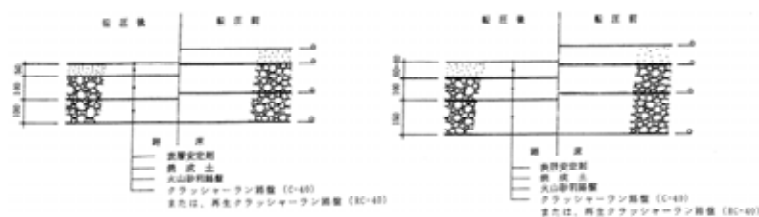
アンツーカー舗装の例【出典：都市公園技術標準解説書（平成22年度版）】
