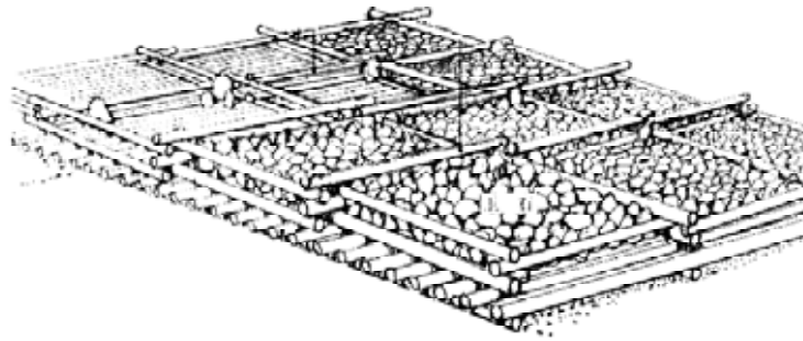
木工沈床の例【出典：多自然型河川工法設計施工要領（案）】
