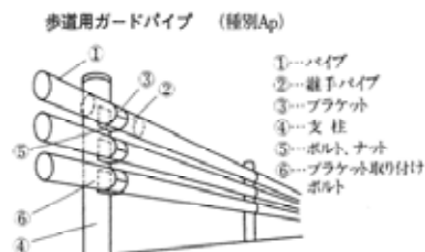
ガードパイプの例【出典：改訂3版土木施工の実際と解説】
