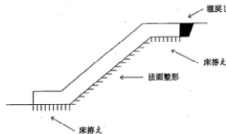
じゃかごの例【出典：土木工事標準積算基準書】
