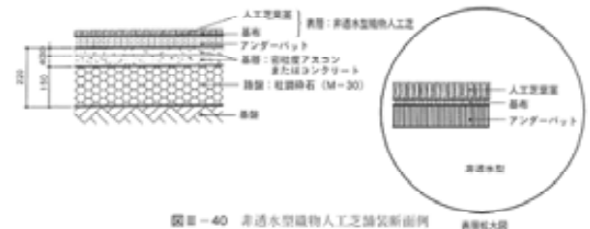
図面-40 非透水性人工芝舗装断面図
