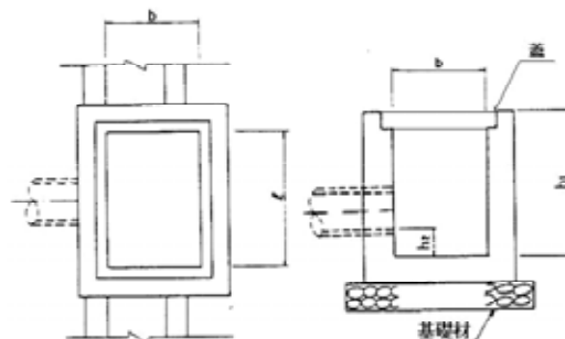
集水樹の例【出典：北陸地方整備局標準設計】
