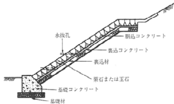
雑割石張の例【出典：道路用語事典】
