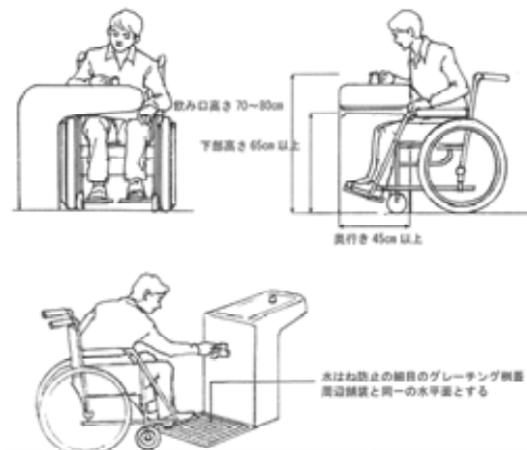
水飲み場の例【出典：都市公園技術標準解説書（平成22年度版）】
