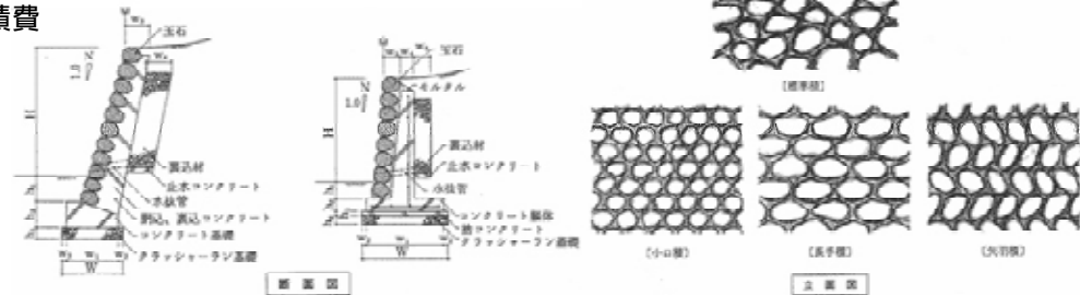
玉石積の例【出典：ランドスケープの修景石工事マニュアル】
