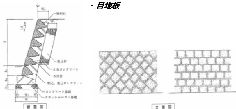
雑割石積の例【出典：ランドスケープの修景石工事マニュアル】
