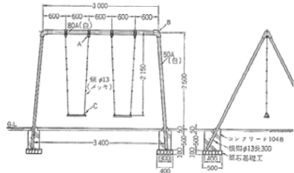
ブランコの例【出典：造園ハンドブック】
