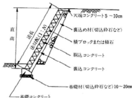
裏込砕石工の例【出典：改訂3版土木施工の実際と解説】
