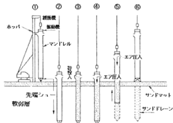
サンドドレーンの施工例【出典：改訂3版土木施工の実際と解説】
