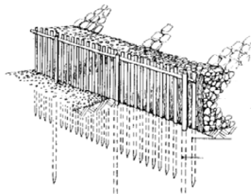
杭柵の例【出典：多自然型河川工法設計施工要領（案）】
