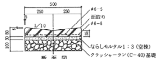
プレキャスト皿型側溝の例
