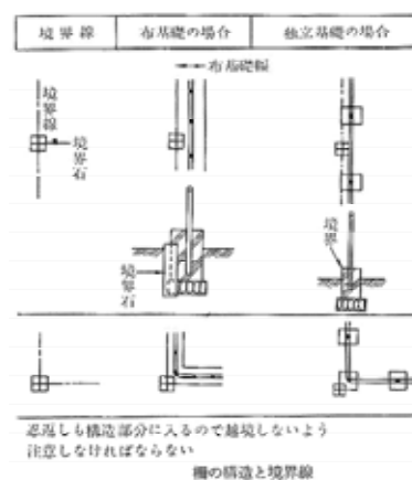
フェンスの例【出典：造園ハンドブック】
