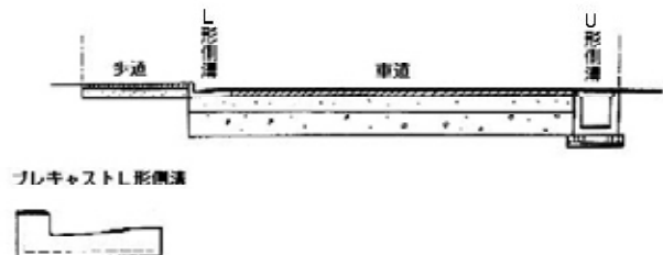
L 型側溝の例【出典：一般土木用語事典】
