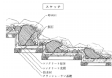
滝石組の例【出典：ランドスケープの修景石工事マニュアル】
