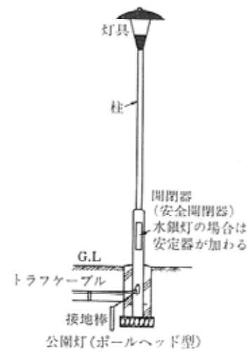
照明灯の例【出典：造園ハンドブック】
