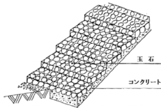
玉石階段の例【出典：多自然型河川工法設計施工要領（案）】
