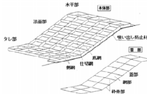
かごマットの例【出典：北陸地方整備局標準設計】
