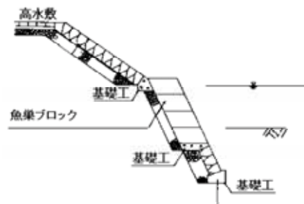
階段ブロック積の例【出典：建設資材ハンドブック】
