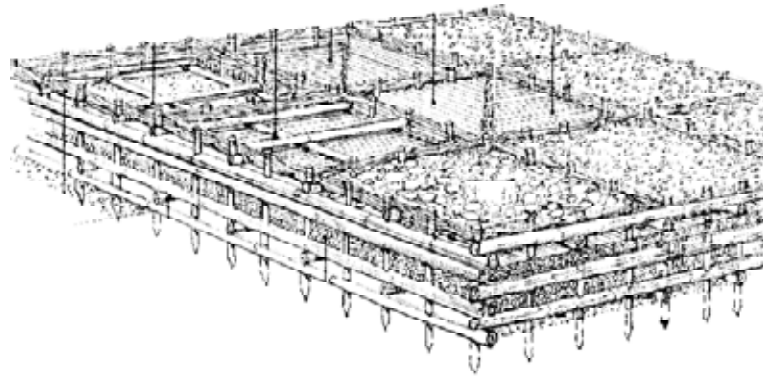
粗朶沈床の例【出典：多自然型河川工法設計施工要領（案）】
