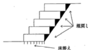
ふとんかごの例【出典：土木工事標準積算基準書】
