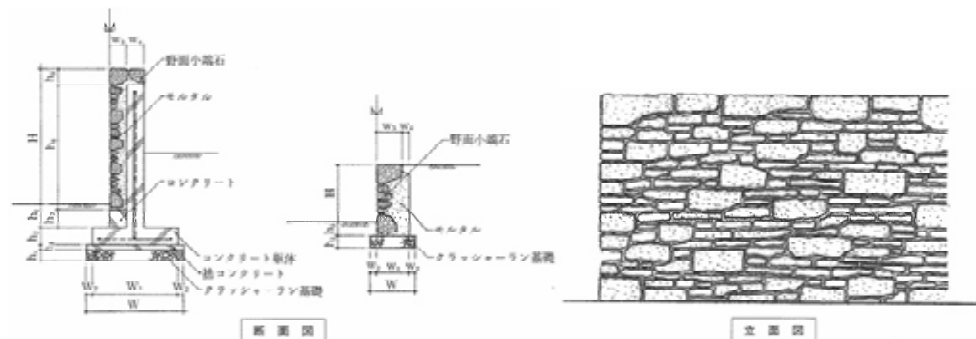
小端積の例【出典：ランドスケープの修景石工事マニュアル】
