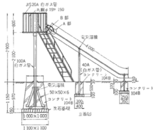
滑台の例【出典：造園ハンドブック】
