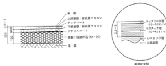
図面-26 アスファルト系舗装断面図例
