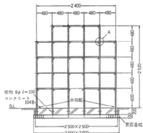
ジャングルジムの例【出典：造園ハンドブック】
