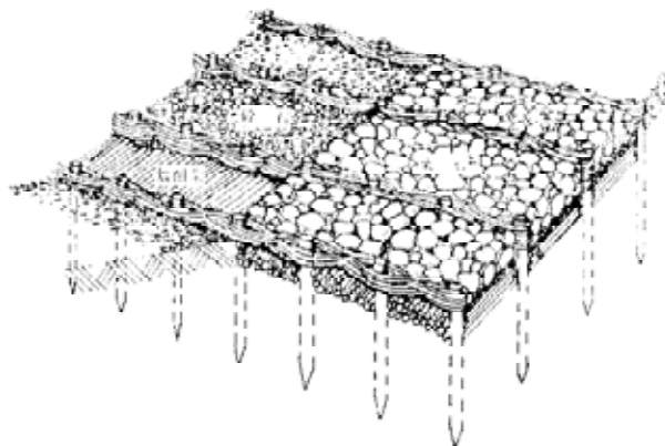
粗朶法覆の例【出典：多自然型河川工法設計施工要領（案）】
