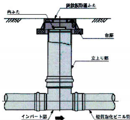
塩化ビニル製樹の例【出典：小型マンホール技術資料プラスチック・マスマンホール協会】
