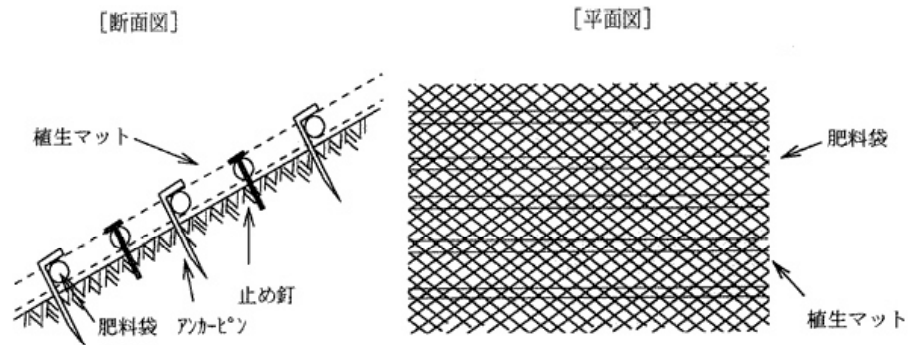
植生マットの例【出典：土木工事標準積算基準書】
