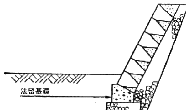
現場打基礎（積み）の例【出典：河川砂防技術基準（案）設計編】
