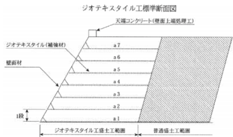
ジオテキスタイル工標準断面図【出典：土木工事標準積算基準書】
