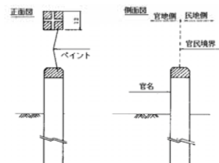
境界杭の例
