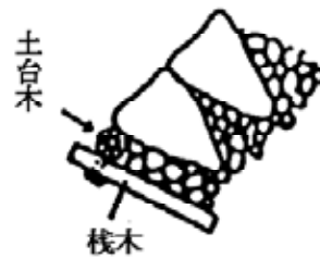
片梯子土台の例【出典：土木工事標準積算基準書】
