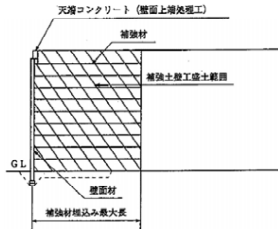
補強土壁の例【出典：土木工事標準積算基準書】
