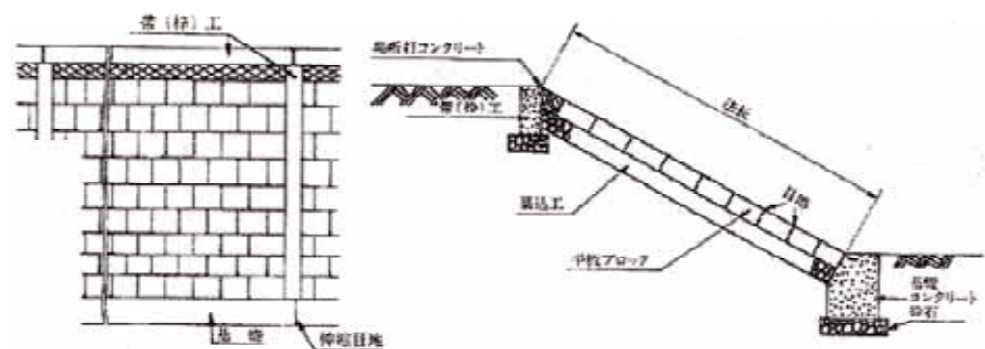
平ブロック張の施工例【出典：改訂3版土木施工の実際と解説】
