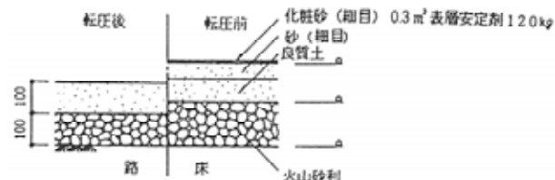
グラウンド・コート砂舗装の例【出典：造園施設設計資料集】
