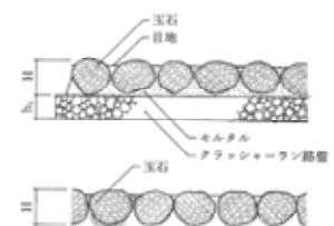
断面図
