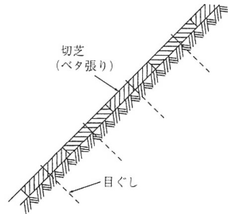
公園張芝の例【出典：道路土工 - のり面工・斜面安定工指針】
