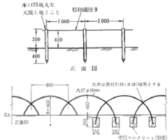
保護柵の例【出典：造園ハンドブック】
