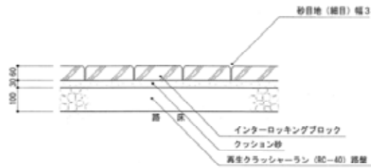
断面図
