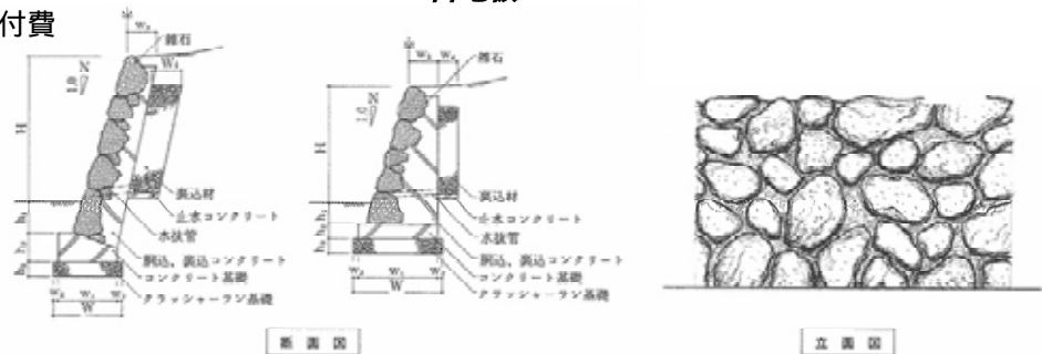
雑石積の例【出典：ランドスケープの修景石工事マニュアル】
