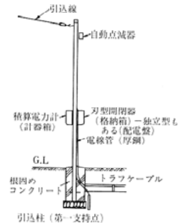
引込柱の例【出典：造園ハンドブック】
