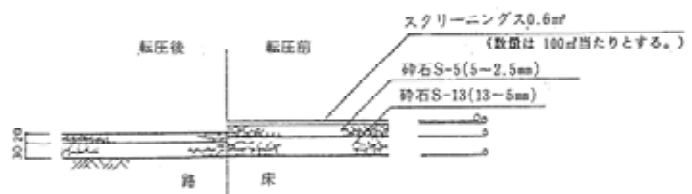
碎石舗装の例【出典：造園施設標準設計図集 平成6年】
