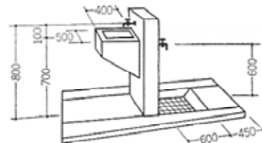
足洗い場の例【出典：造園ハンドブック】
