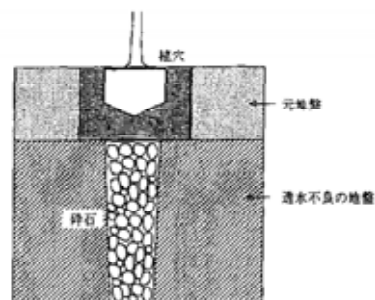
縦穴排水の例【出典：都市公園技術標準解説書（平成22年度版）】
