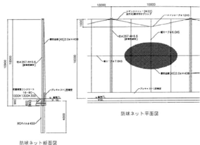
防球ネットの例【出典：都市公園技術標準解説書（平成22年度版）】
