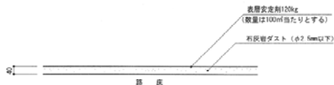
石灰岩ダスト舗装の例【出典：造園施設標準設計図集 平成19年】
