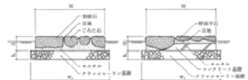
断面図
