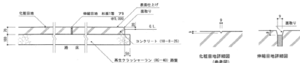
断面図
