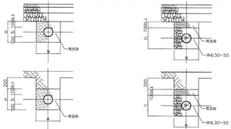
暗渠排水の例【出典：都市公園技術標準解説書（平成22年度版）】
