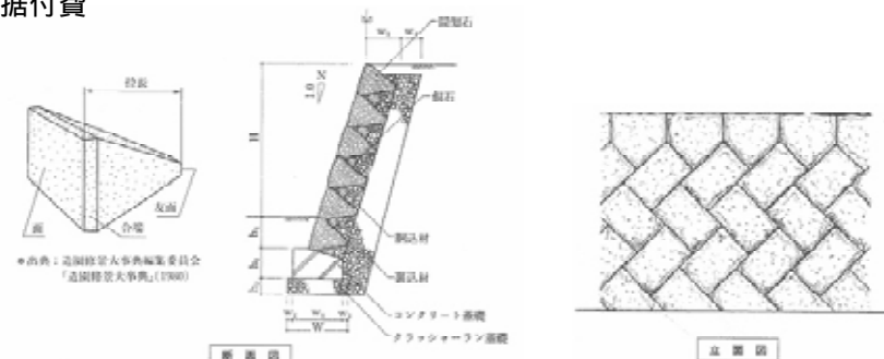
間知石積の例【出典：ランドスケープの修景石工事マニュアル】
