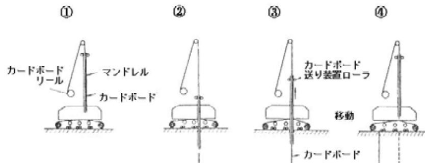
ペーパードレーンの施工例【出典：道路土工・軟弱地盤対策工指針】
