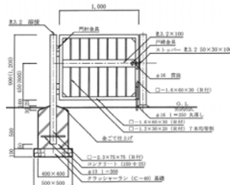
門扉の例【出典：撤去・移設等標準設計図集】
