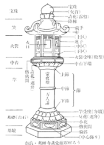
灯籠の例【出典：造園ハンドブック】
