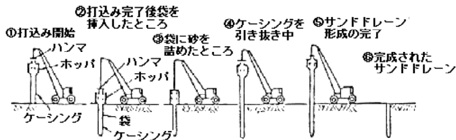
袋詰式サンドドレーンの施工例【出典：道路土工・軟弱地盤対策工指針】
