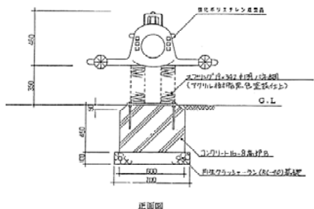
スプリング遊具の例
