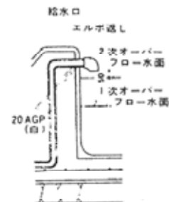
吐出口の例【出典：住宅団地の造園施設】
