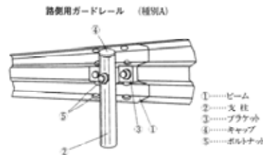
ガードレールの例【出典：改訂3版土木施工の実際と解説】
