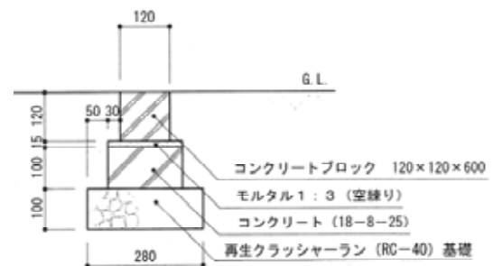
舗装止めの例【出典：造園施設標準設計図集 平成19年】
