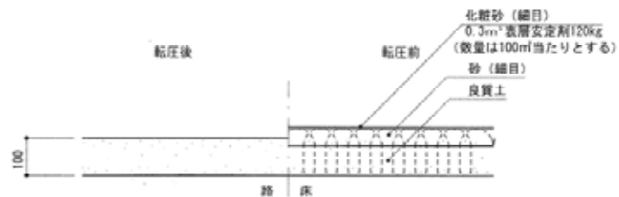
砂舗装の例【出典：造園施設標準設計図集 平成19年】
