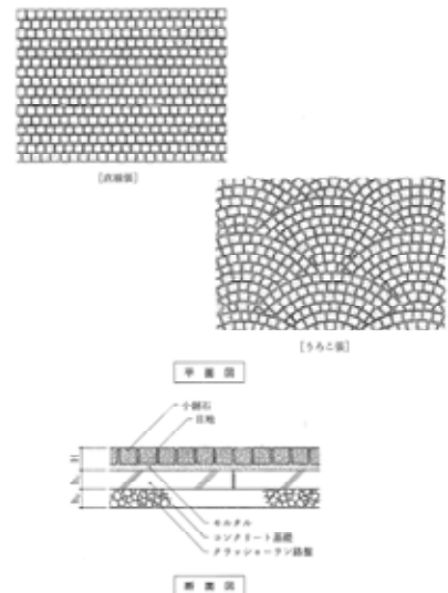
小舗石舗装の例【出典：ランドスケープの修景石工事マニュアル】
