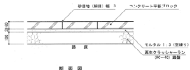
断面図 平板舗装の例【出典：造園施設標準設計図集 平成19年】
