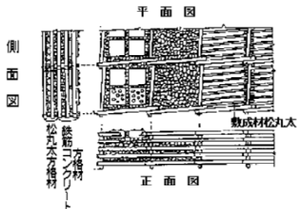
改良沈床の例【出典：河川・ダム・砂防用語事典】
