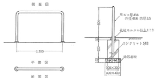
車止めの例【出典：造園ハンドブック】
