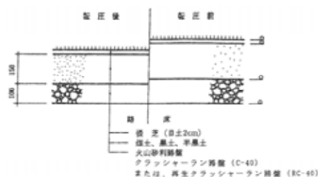
天然芝舗装の例【出典：都市公園技術標準解説書（平成22年度版）】
