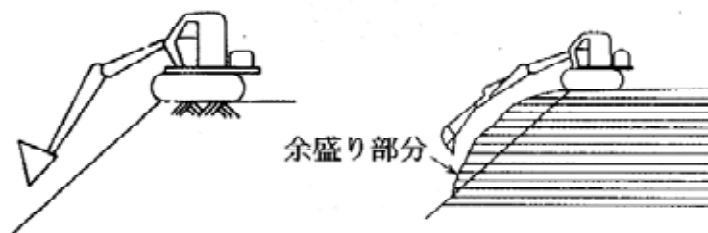
法面整形（盛土部）の施工例【出典：改訂3版土木施工の実際と解説】
