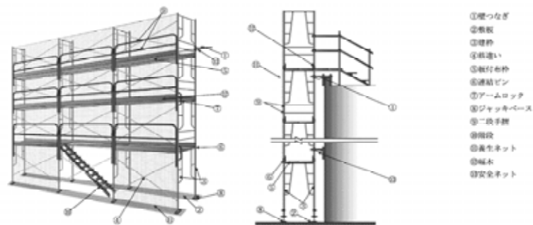
手摺先行型枠組足場の組立例
