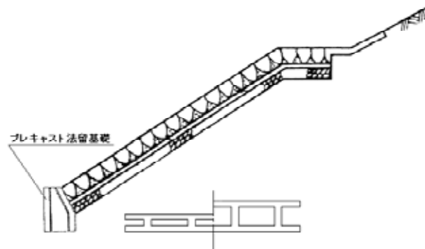
プレキャスト基礎の例【出典：道路用語事典、北陸地方整備局標準設計】
