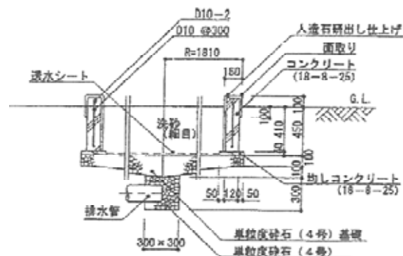
砂場の例【出典：都市公園技術標準解説書（平成22年度版）】
