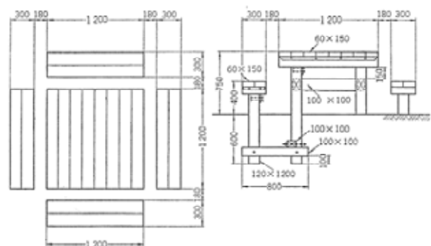
野外卓の例【出典：造園ハンドブック】
