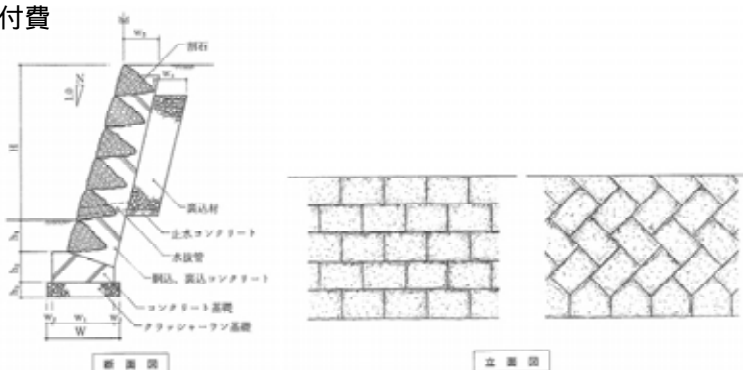
割石積の例【出典：ランドスケープの修景石工事マニュアル】
