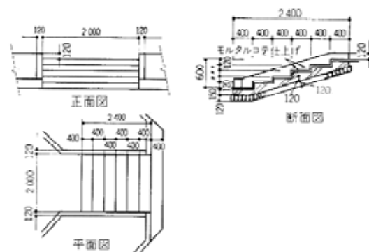
コンクリート階段の例【出典：造園ハンドブック】
