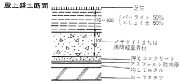
人工地盤客土の例【出典：ディテール17】
