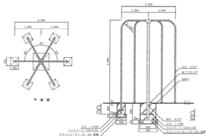
はん登棒の例【出典：撤去・移設等標準設計図集】
