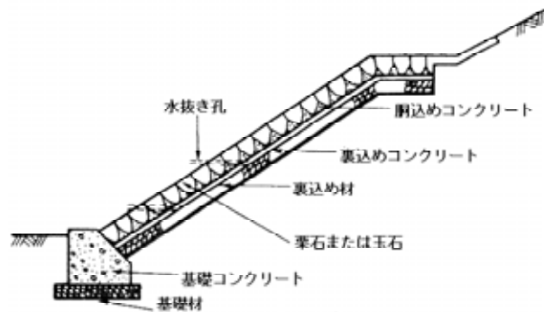
石張の例【出典：道路用語事典】
