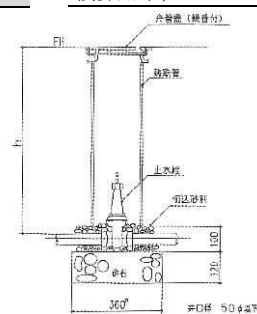
止水栓の例
