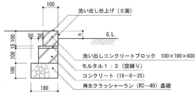
擬石縁石の例【出典：造園施設標準設計図集平成 19 年】
