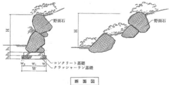
崩れ積の例【出典：ランドスケープの修景石工事マニュアル】
