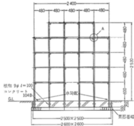
ジャングルジムの例【出典：造園ハンドブック】
