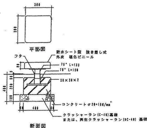
塁ベースの例【出典：都市公園技術標準解説書（平成22年度版）】
