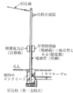
引込柱の例【出典：造園ハンドブック】
