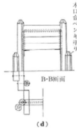
解説板の例【出典：造園ハンドブック】
