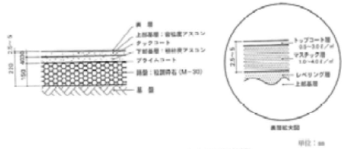
図面-26 アスファルト系舗装断面図例
