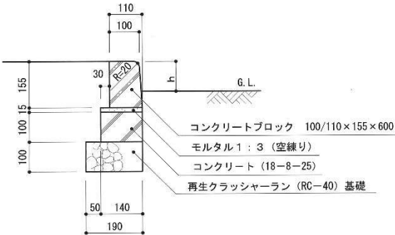
コンクリート縁石の例【出典：造園施設標準設計図集平成19年】
