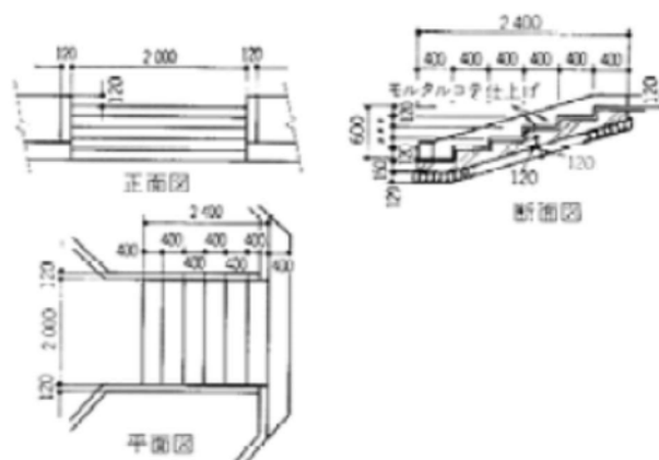
コンクリート階段の例【出典：造園ハンドブック】
