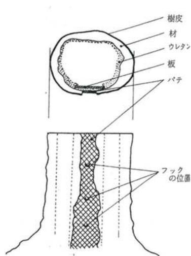
内部の空洞部のウレタンによる 修復参考例【出典：新・樹木医の手引き】
