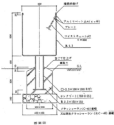
くず入れの例【出典：造園施設標準設計資料集】
