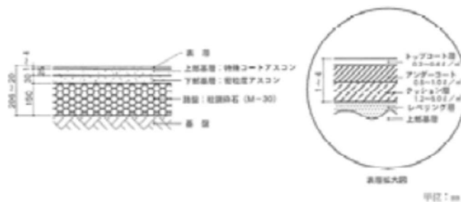
図29 アスファルト樹脂系舗装断面図
