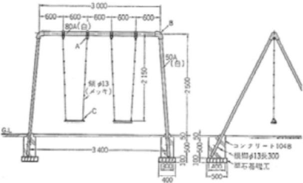
ブランコの例【出典：造園ハンドブック】
