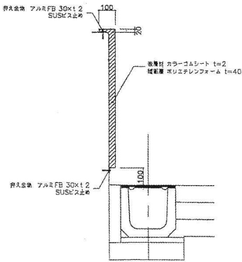
衝撃吸収材の例【出典：都市公園技術標準解説書（平成 22 年度版）】
