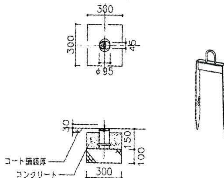
センターガイドの例【出典：都市公園技術標準解説書（平成22年度版）】
