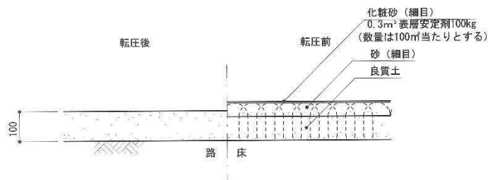
砂舗装の例【出典：造園施設標準設計図集平成 19 年】
