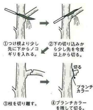
枝降ろしの技法
