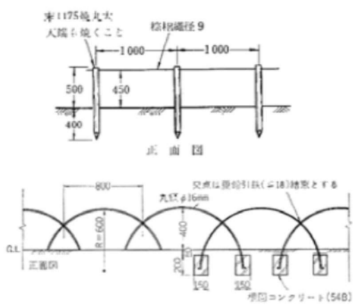
保護柵の例【出典：造園ハンドブック】
