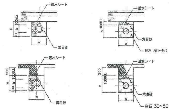
暗渠排水の例【出典：都市公園技術標準解説書（平成 22 年度版）】
