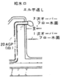
吐出口の例【出典：住宅団地の造園施設】
