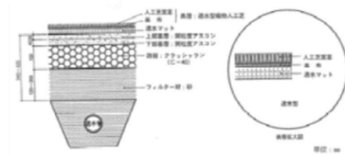
図41 透水型枠物人工芝舗装断面図
