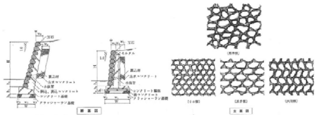
玉石積の例【出典：ランドスケープの修景石工事マニュアル】
