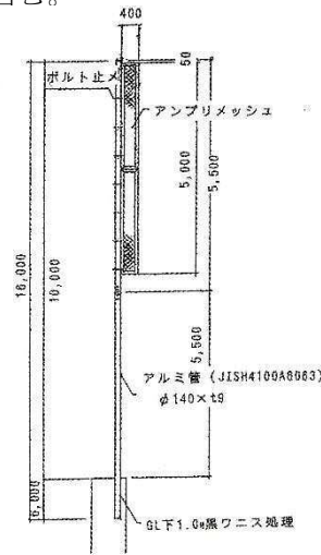
フェールポールの例【出典：都市公園技術標準解説書（平成22年度版）】
