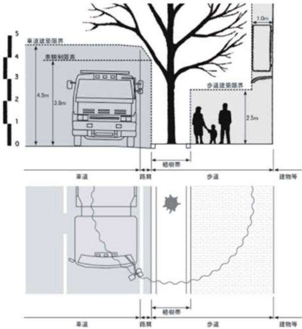
各種制限高と越境枝
