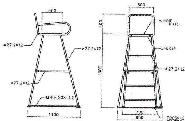
審判台の例【出典：都市公園技術標準解説書（平成22年度版）】
