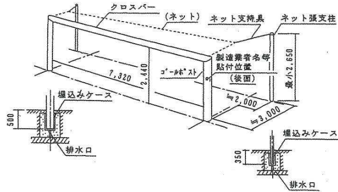
ゴールポストの例【出典：都市公園技術標準解説書（平成22年度版）】
