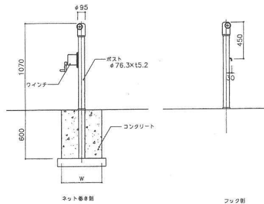
ポストの例【出典：都市公園技術標準解説書（平成22年度版）】
