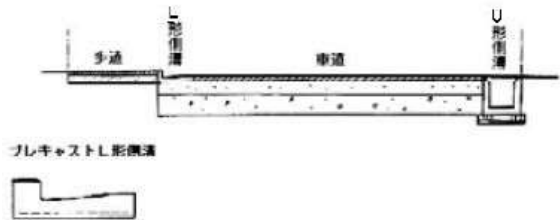
L型側溝の例【出典：一般土木用語事】
