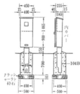
分電盤の例【出典：造園ハンドブック】
