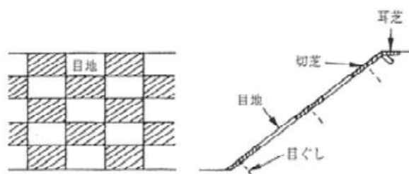
公園市松芝の例【出典：改訂土木施工の実際と解説】
