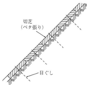
公園張芝の例【出典：道路土工のり面工・斜面安定工指針】
