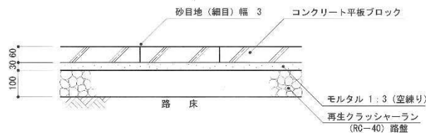
平板舗装の例【出典：造園施設標準設計図集平成 19 年】
