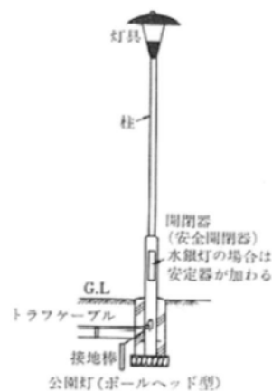
照明灯の例【出典：造園ハンドブック】
