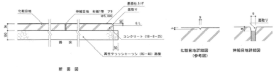
公園コンクリート舗装の例【出典：造園施設標準設計図集平成19年】
