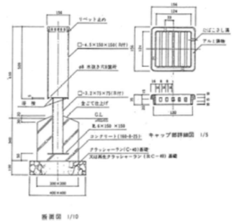
吸殻入れの例【出典：造園施設標準設計資料集】
