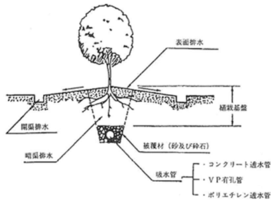
開渠排水の例【出典：監督必携】
