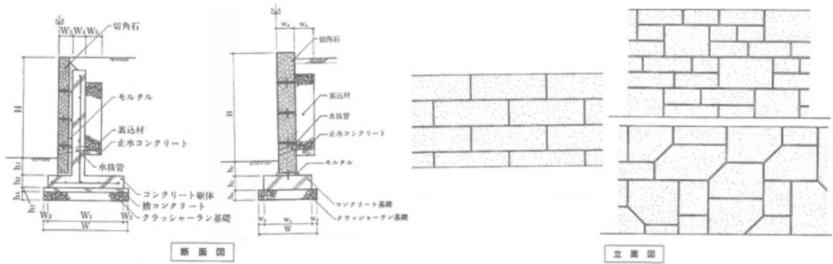
切石積の例【出典：ランドスケープの修景石工事マニュアル】
