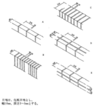
レンガ縁石の例【出典：公園緑地工事標準歩掛】
