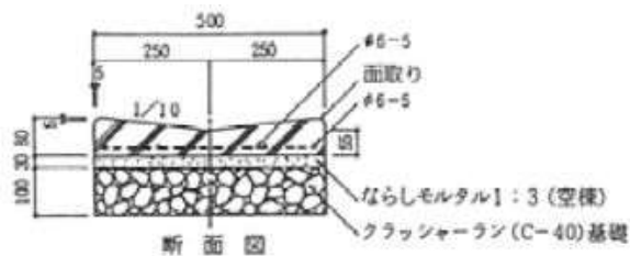
プレキャスト皿型側溝の例
