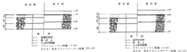
アンツーカー舗装の例【出典：都市公園技術標準解説書（平成 22 年度版）】
