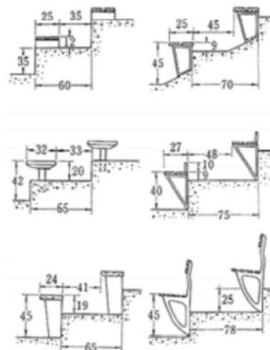
スタンドベンチの例【出典：造園ハンドブック】
