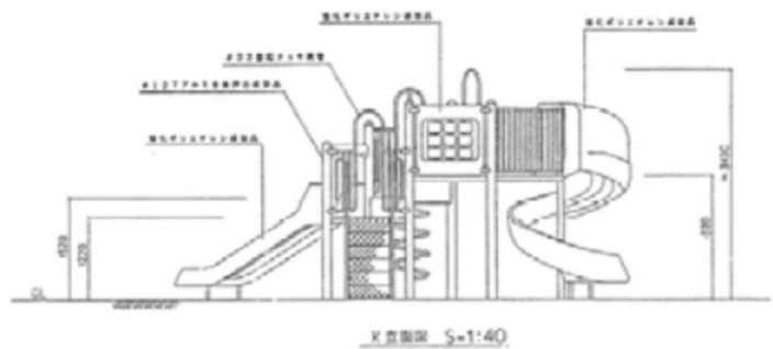
複合遊具の例
