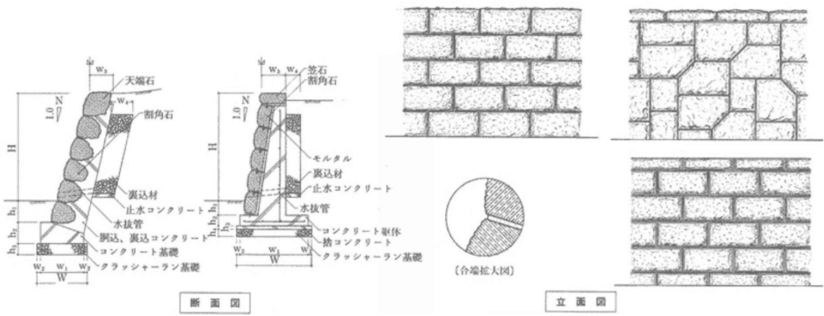
こぶだし石積の例【出典：ランドスケープの修景石工事マニュアル】
