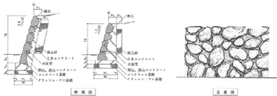
雑石積の例【出典：ランドスケープの修景石工事マニュアル】
