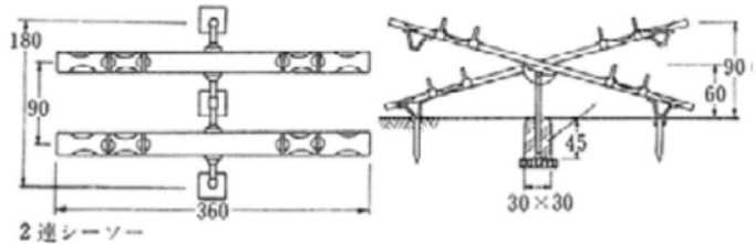
シーソーの例【出典：造園ハンドブック】
