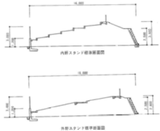
スタンド擁壁の例【出典：屋外体育施設の建設指針平成 17 年改訂版】
