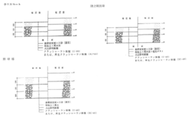
クレー舗装の例【出典：都市公園技術標準解説書（平成22年度版）】
