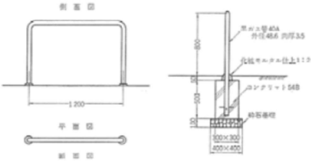
車止めの例【出典：造園ハンドブック】
