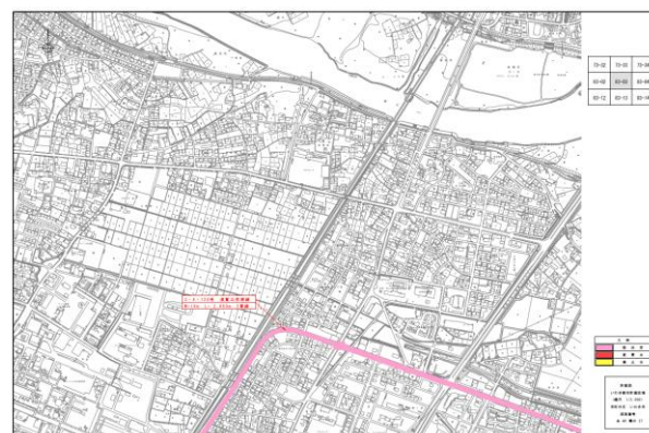
計画図③（須賀三枚笹線）
