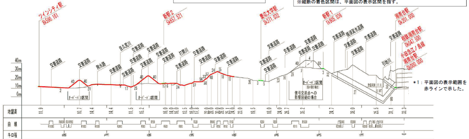
図 平面・縦断計画図計画図：慶応大学～ツインシティ駅間
