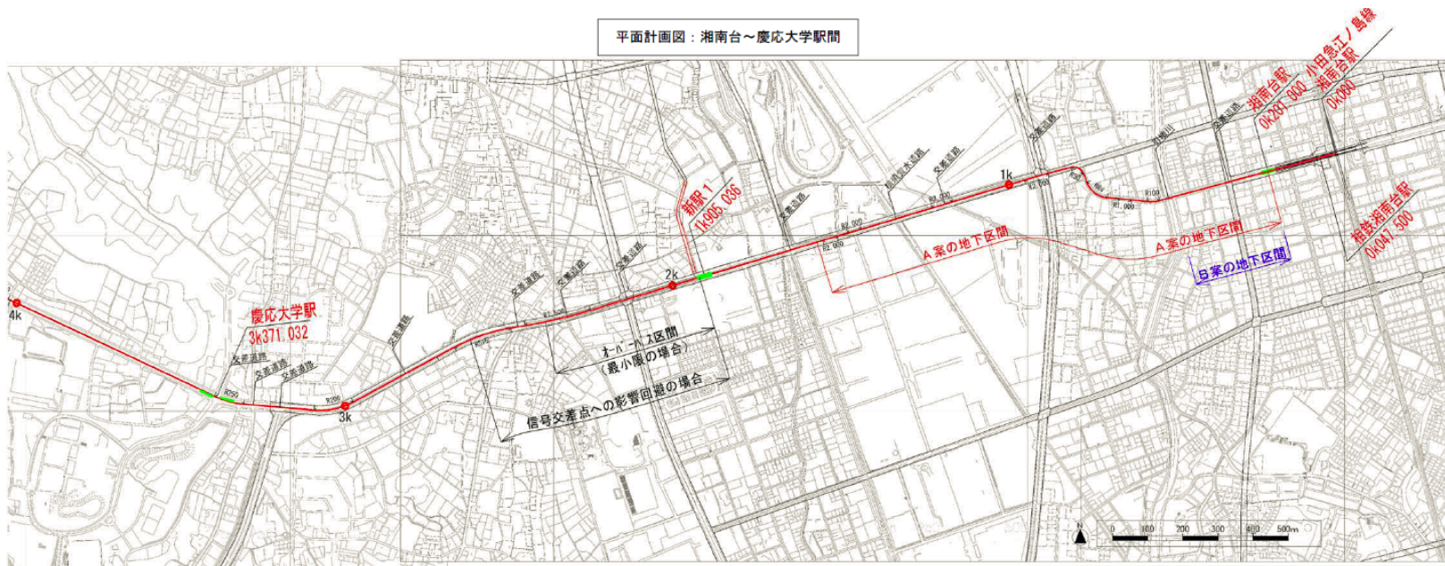
縦断計画図：湘南台～ツインシティ駅間
