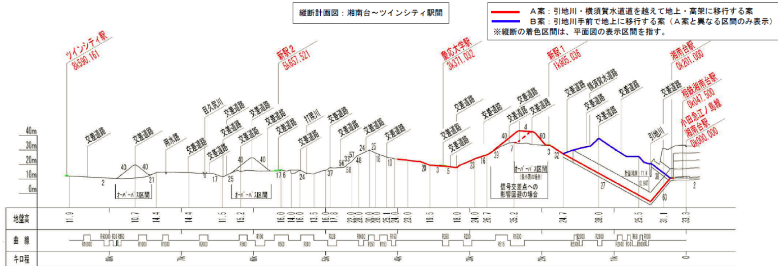
図 平面・縦断計画図：湘南台～慶応大学駅間
