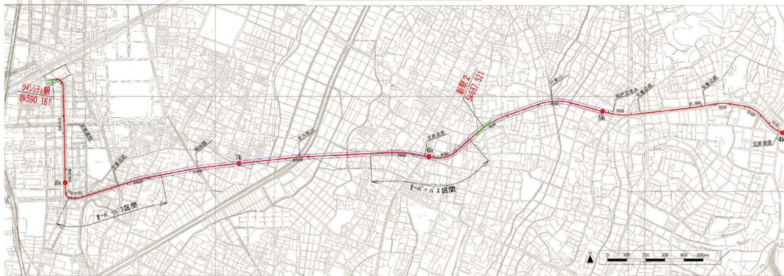
縦断計画図：湘南台～ツインシティ駅間
