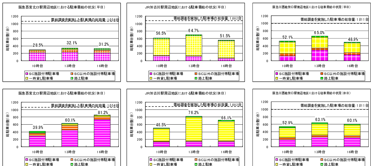
図 2－10 3地区の地区全体での駐車需給バランス
