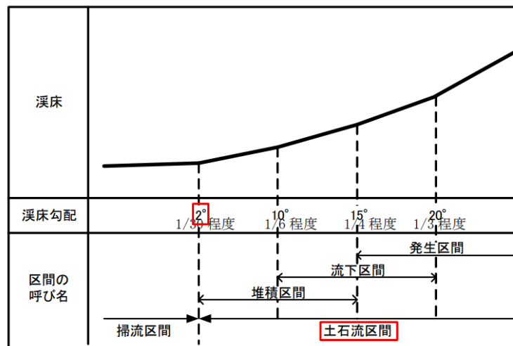
図 5.8 土砂移動の形態の溪床勾配による目安
