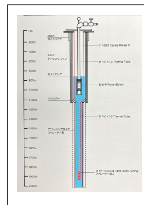
二重ケーシング工法
