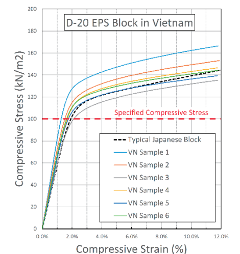
ベトナム製造 EPS ブロックの圧縮試験例
