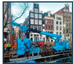
オランダ・アムステルダム護岸改修
