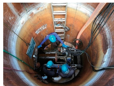
液状化対策工事（GM 推進工）
