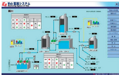
▲制御監視システム
