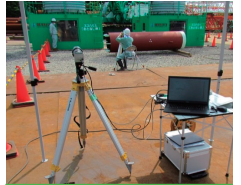
サンプリングモアレカメラと 制御・記録・作図用 P C
