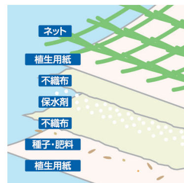
提案製品の構造
