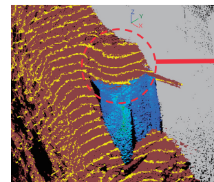
3D ソナーで除去前を確認
