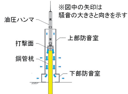
騒音防止装置 エコハウス「おとなし君」
