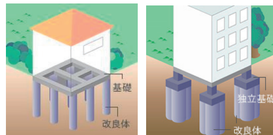
低層建築物の基礎
