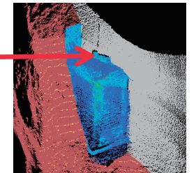
3D ソナーで除去後を確認
