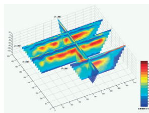
水源調査 3D 解析(物理探査)
