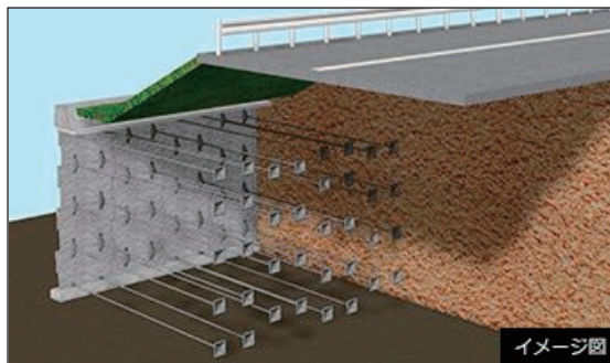
多数アンカー式補強土壁工法
