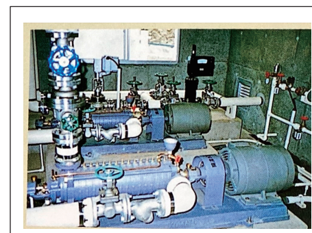
温泉設備工事ポンプ室 湯ヶ島高原クラブ
