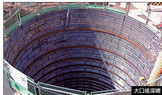
深礎杭（ライナープレート）
