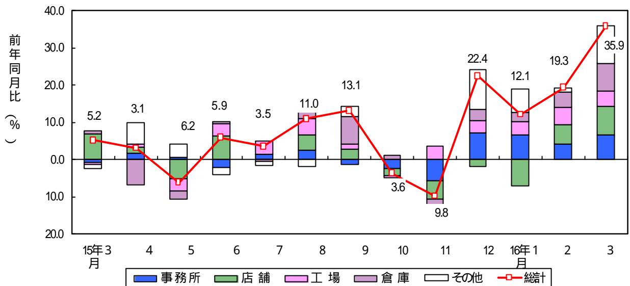
民間非居住用建築物着工床面積の伸びと使途別寄与度
