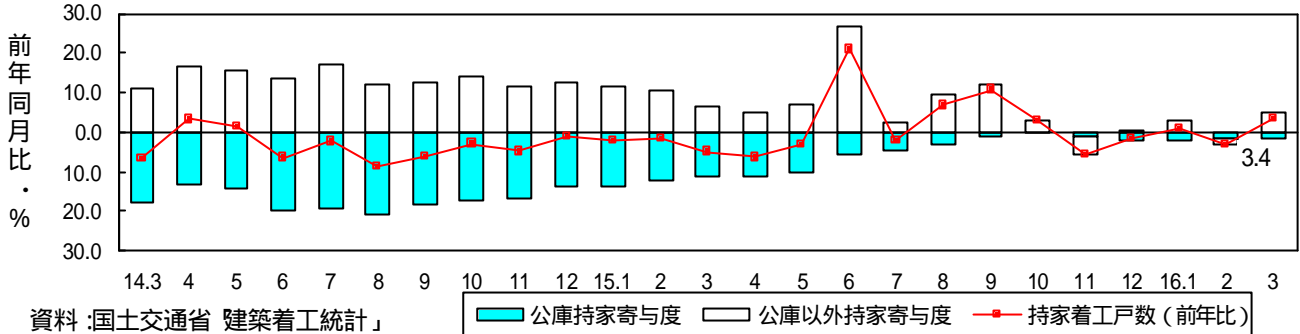
持家着工と資金別寄与度の推移
