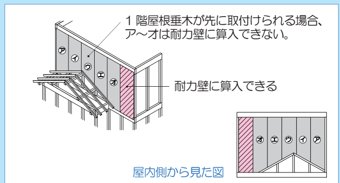
耐力壁と認められない場合の例
